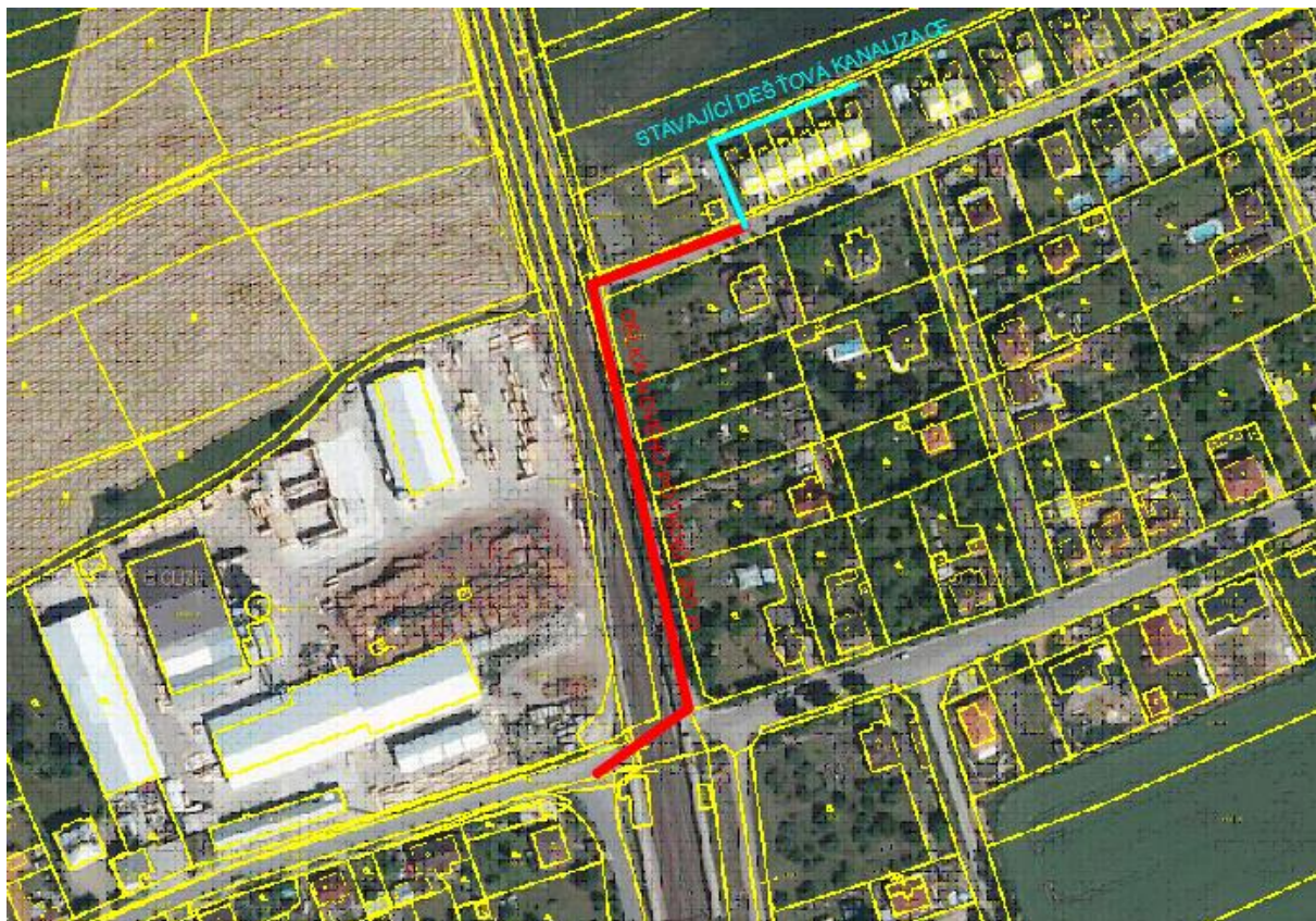
Obr. 7 MP 8 - Výstavba nového potrubí
