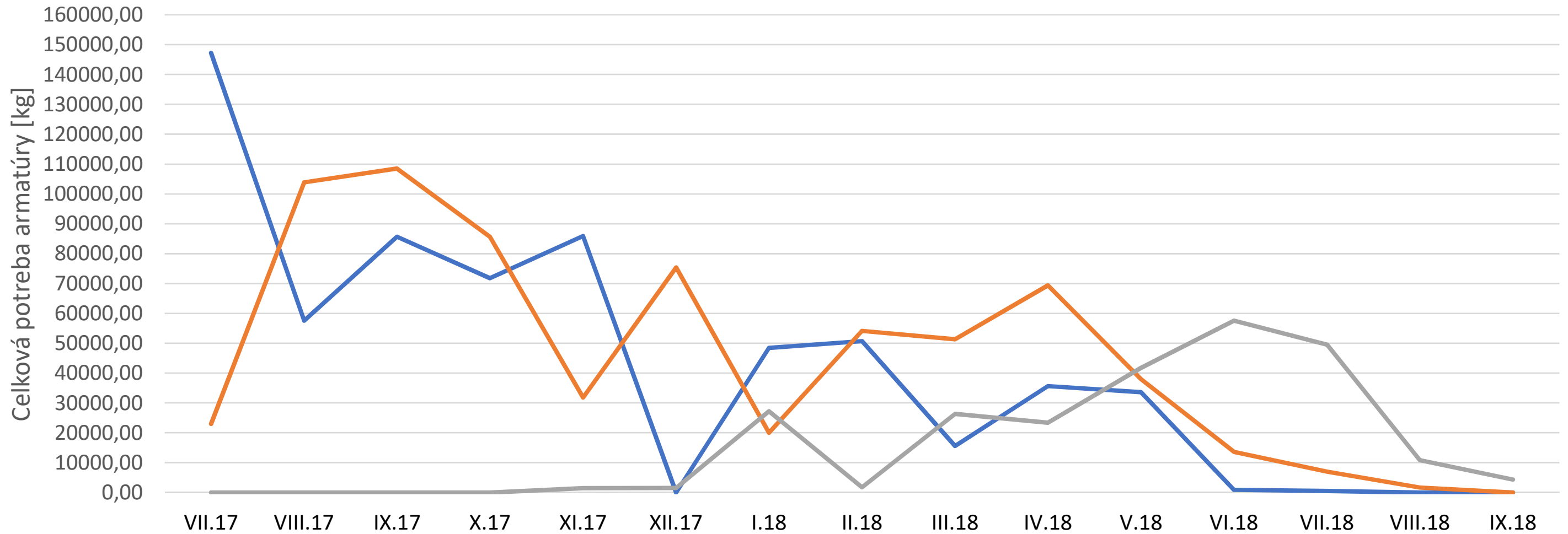
Graf potreby armatúry v čase - Biologická vodná linka - L4
