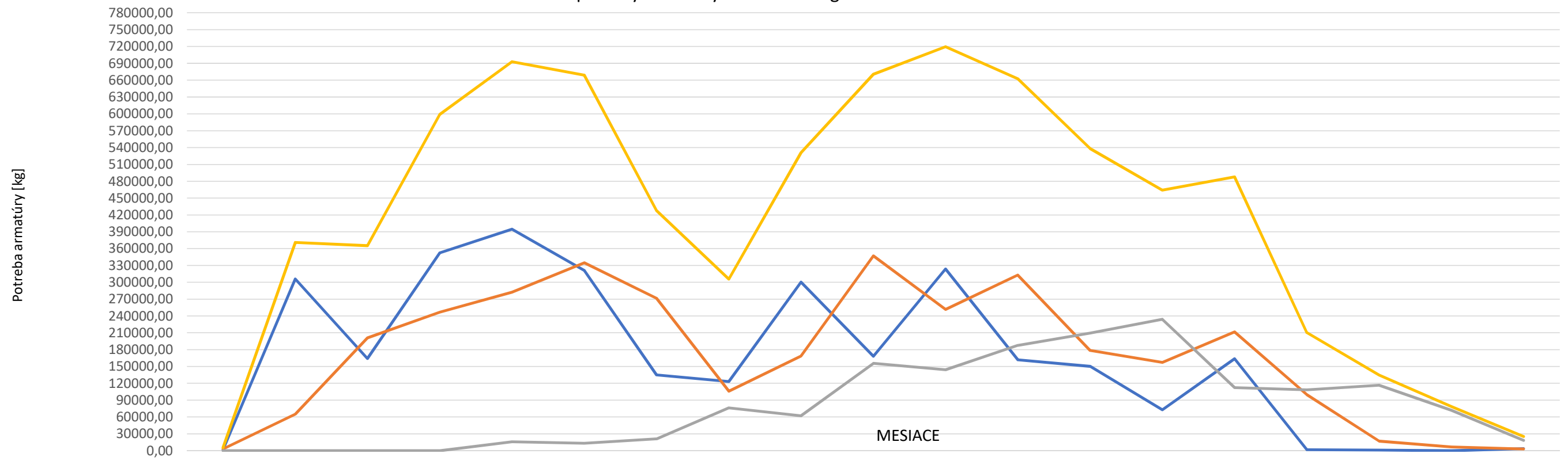
Graf potreby armatúry v čase - Biologická vodná linka - KOMPLET
