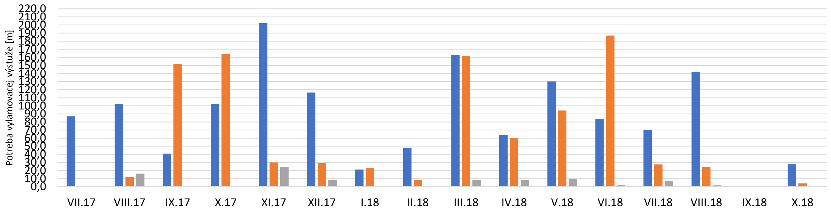
Graf potreby vylamovacej výstuže - Biologická vodná linka - KOMPLET
