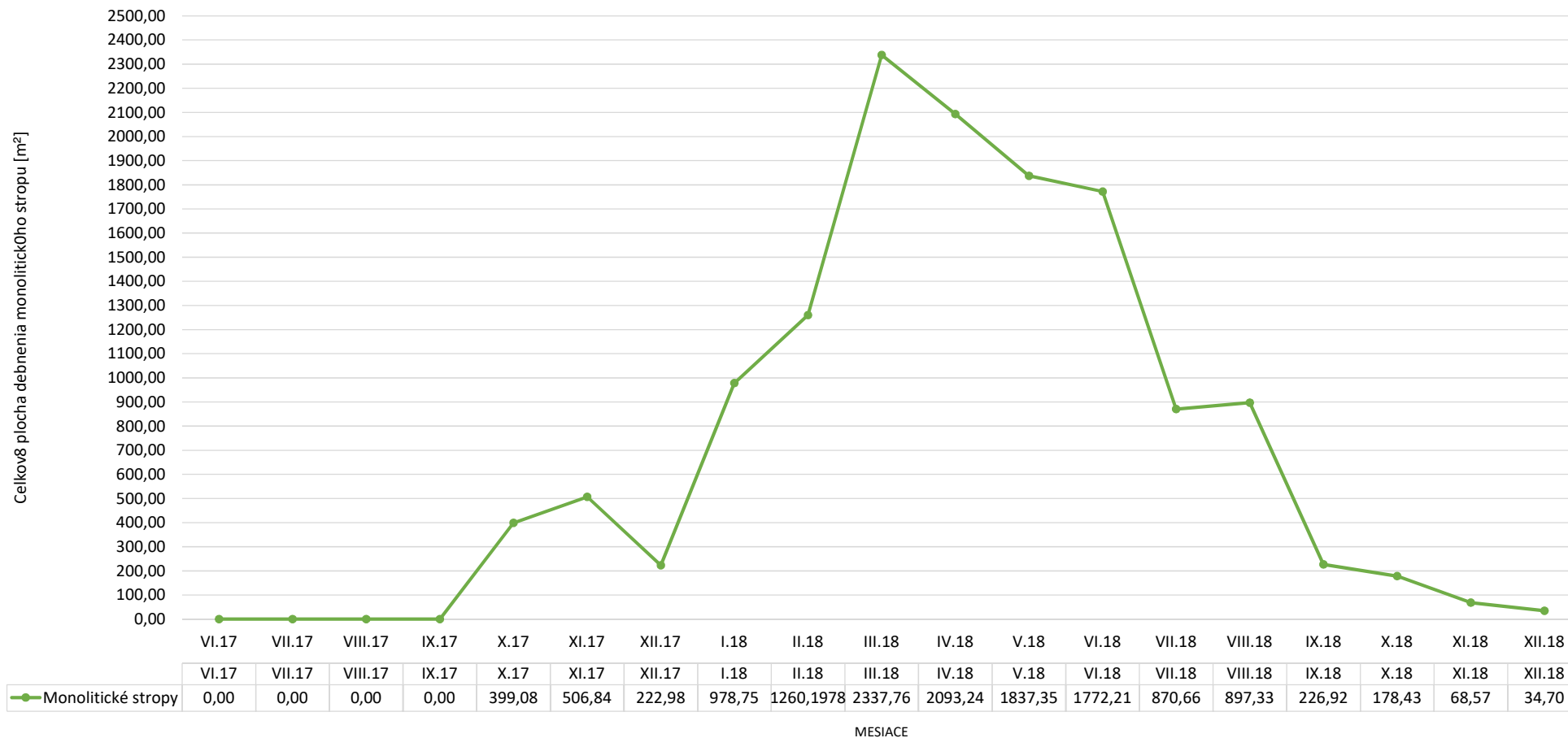
Graf debnenia monilitického stropu - práca - Biologická vodná linka - KOMPLET
