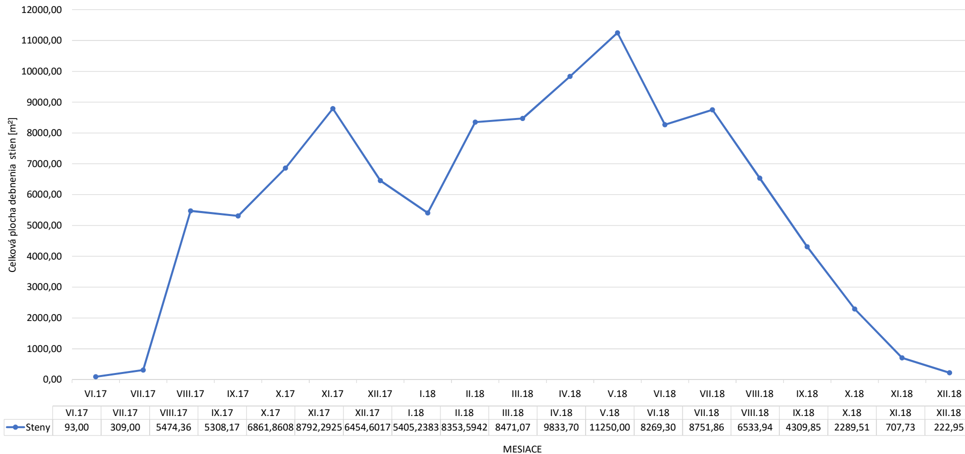
Graf debnenia stien - práca - Biologická vodná linka - KOMPLET
