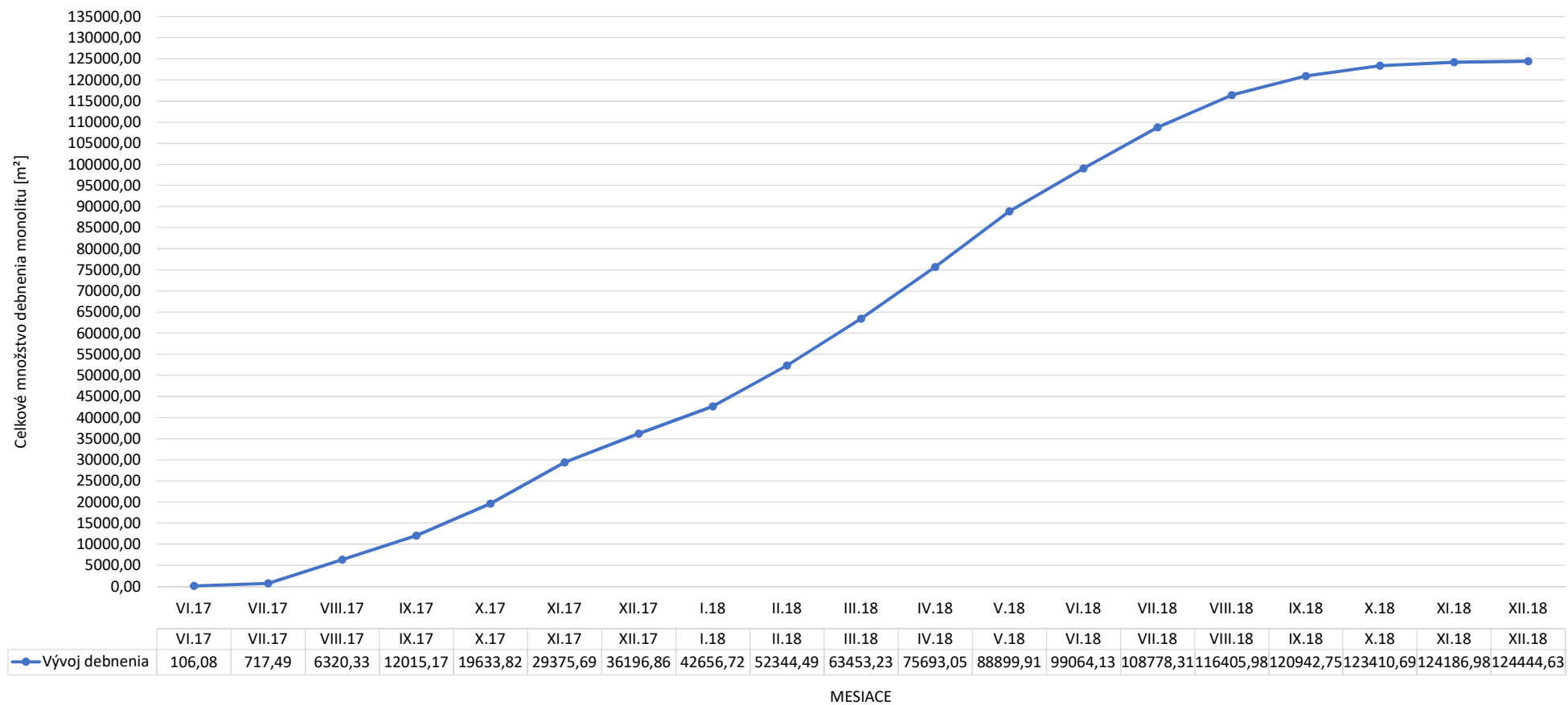
Graf kontroly stavu debnenia monolitu - Biologická vodná linka - KOMPLET
