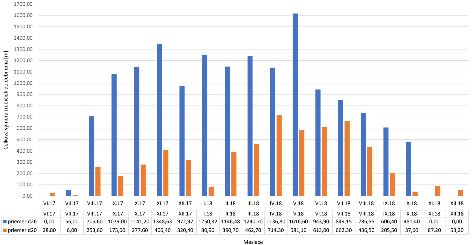
Graf potreby trubičiek do debnenia - Biologická vodná linka - KOMPLET
