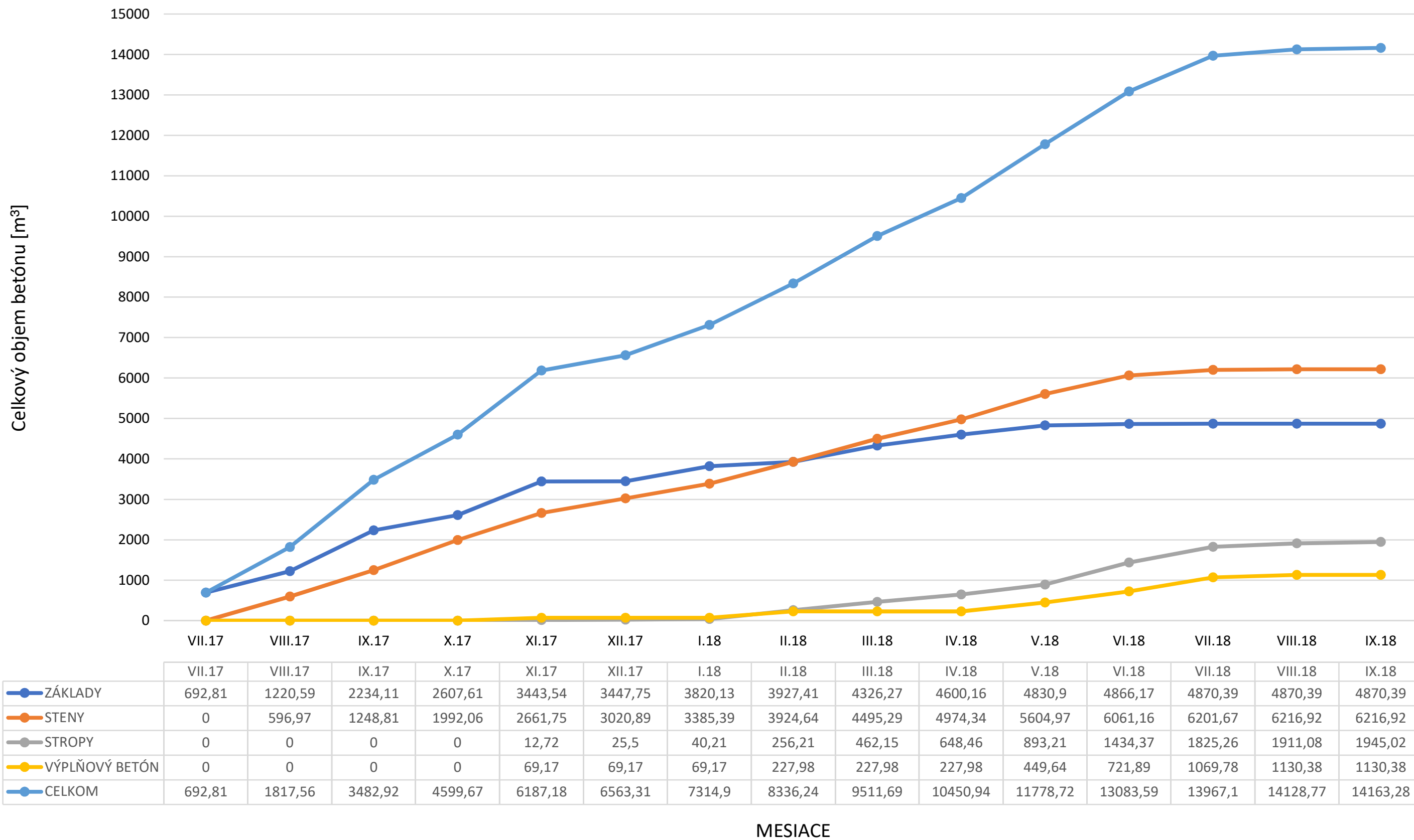
Graf vytvorenej hodnoty v čase - Biologická vodná linka - LINKA 4
