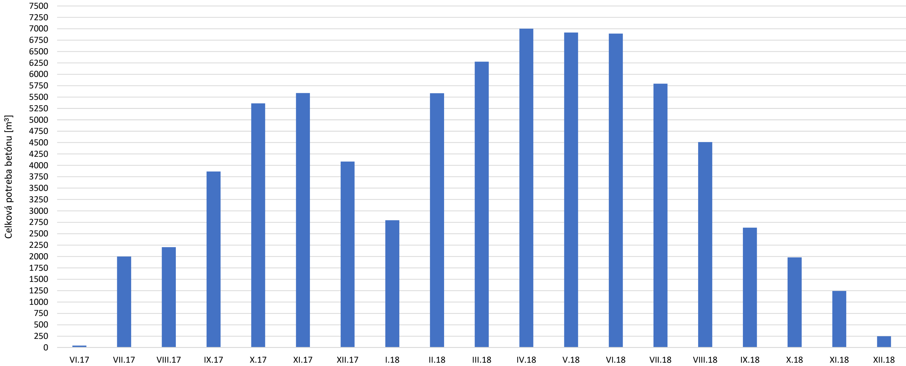
Graf potreby betónu - Biologická vodná linka - KOMPLET
