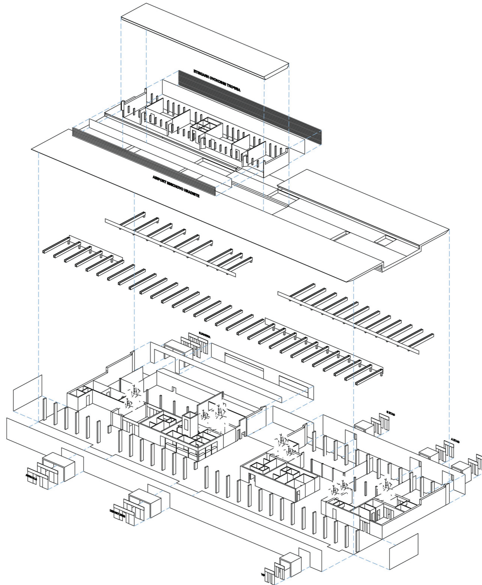
A6 - KONŠTRUKČNÁ SCHÉMA
