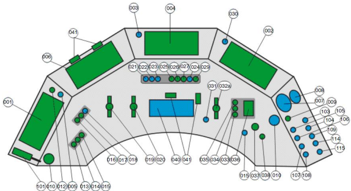
Obr. 1 – Standardizovaný řídicí pult strojvedoucího elektrických ucelených jednotek (Electric Multiple Unit, EMU)/ dieselových ucelených jednotek (Diesel Multiple Unit, DMU), lokomotiv and řídicích vozů
