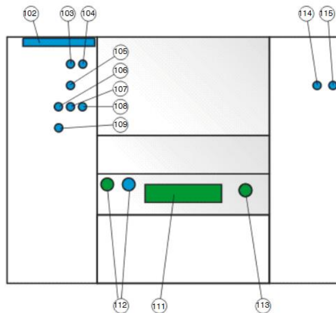
Obr. 2 – Standardizovaný řídicí pult strojvedoucího elektrických ucelených jednotek (Electric Multiple Unit, EMU)/ dieselových ucelených jednotek (Diesel Multiple Unit, DMU), lokomotiv and řídicích vozů
