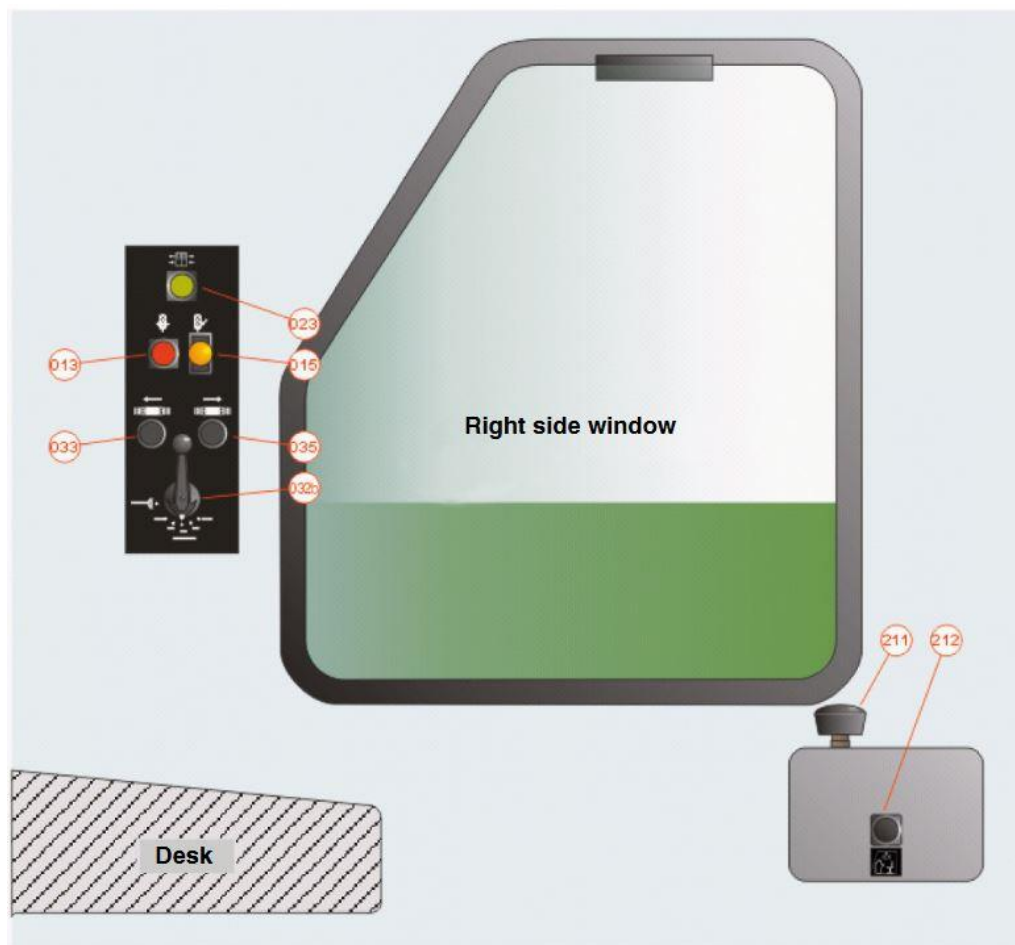
Obr. 3 – Příklad pomocného stolku strojvedoucího na boční stěně kabiny strojvedoucího
