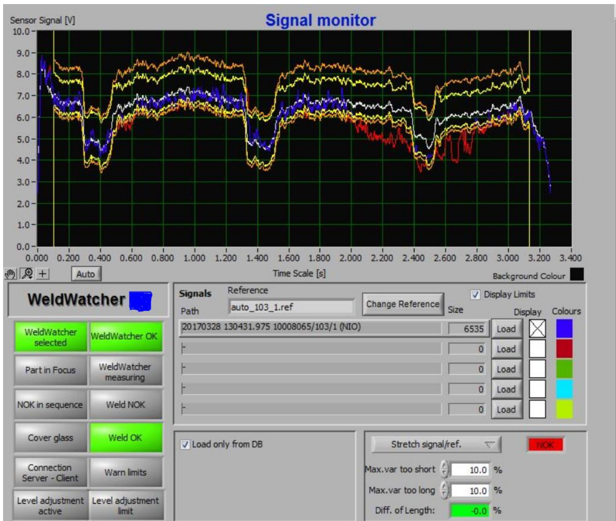
Příloha 15: vzorek 30, svar 24, Weld watcher
