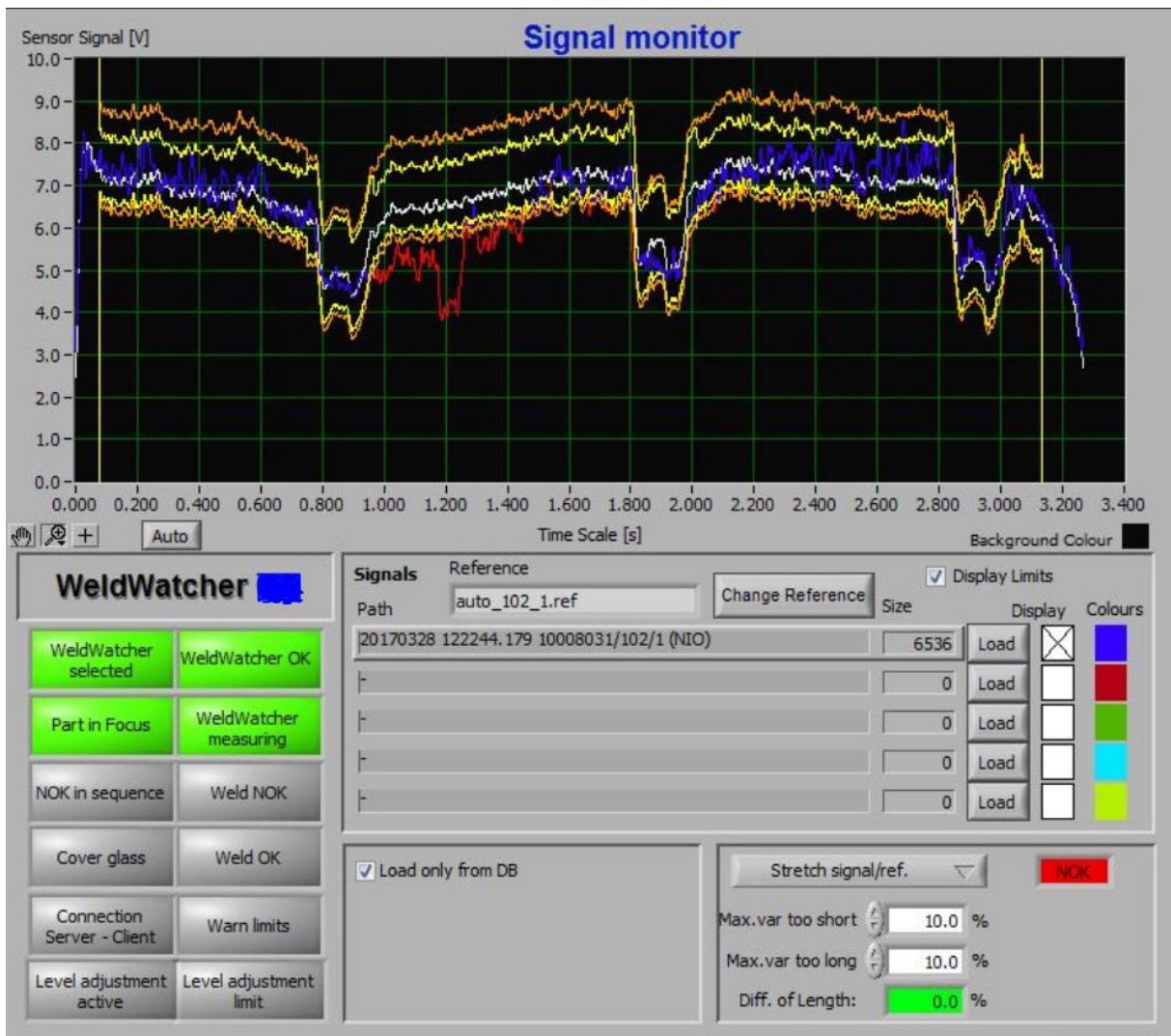
Příloha 5: vzorek 4, svar 23, Weld watcher
