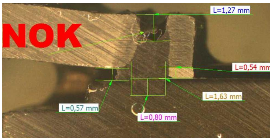
Příloha 9: vzorek 27, svar 23, řez 2
