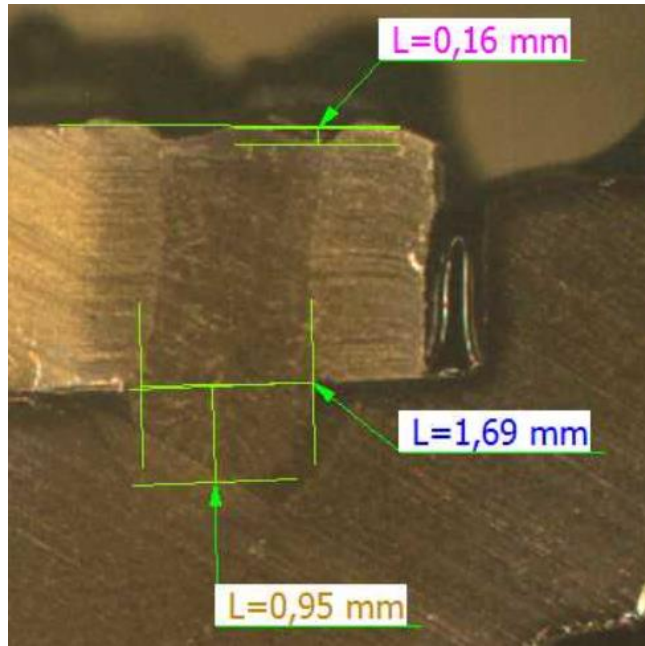
Příloha 7: vzorek 27, svar 23, řez 3
