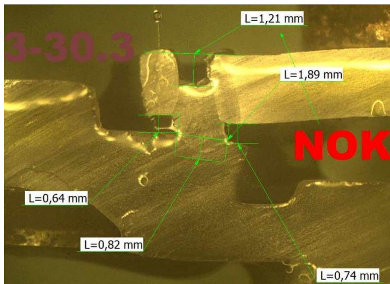
Příloha 14: vzorek 30, svar 24, řez 3
