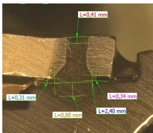
Příloha 2: vzorek 4, svar 23, 1. řez
