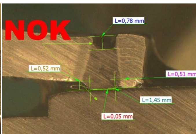
Příloha 3: vzorek 4, svar 23, 2. řez
