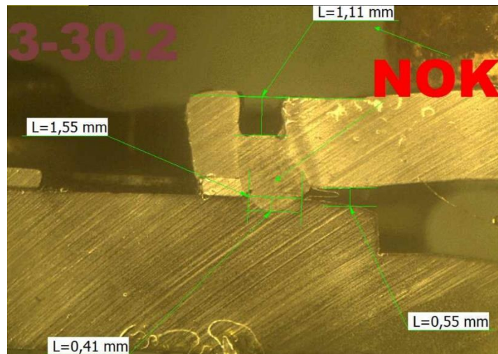
Příloha 13: vzorek 30, svar 24, řez 2
