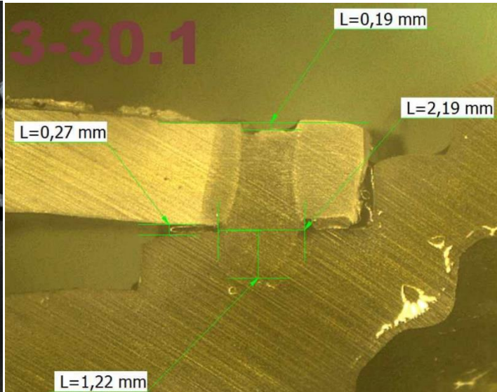
Příloha 12: vzorek 30, svar 24, řez 1
