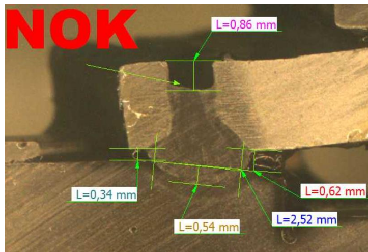
Příloha 8: vzorek 27, svar 23, řez 1
