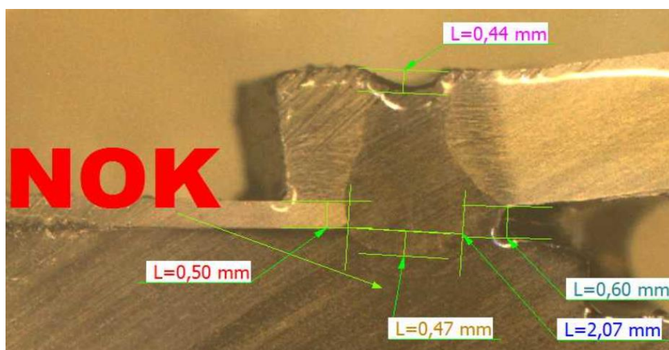
Příloha 4: vzorek 4, svar 23, 3. řez
