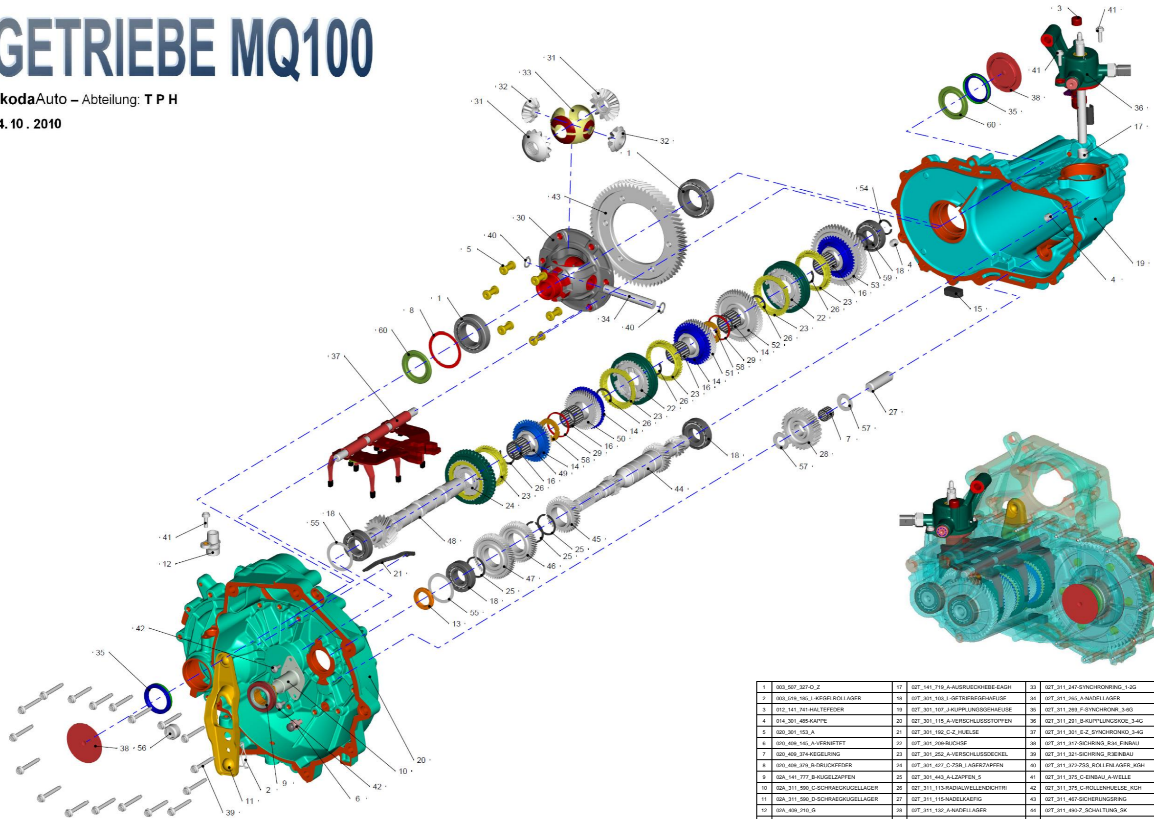
Příloha 4: Rozklad převodovky MQ 100 [4]
