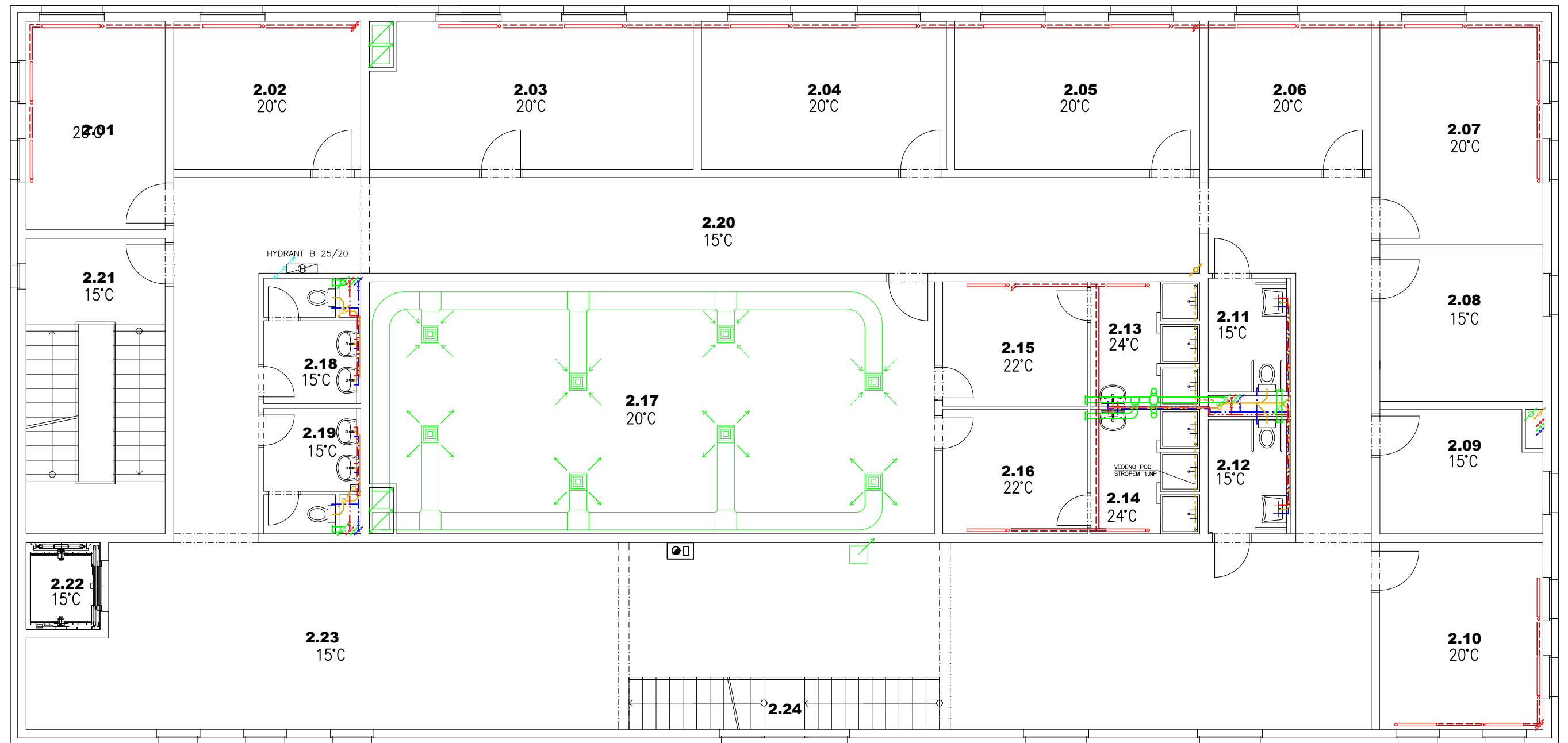
TABULKA MÍSTNOSTÍ
