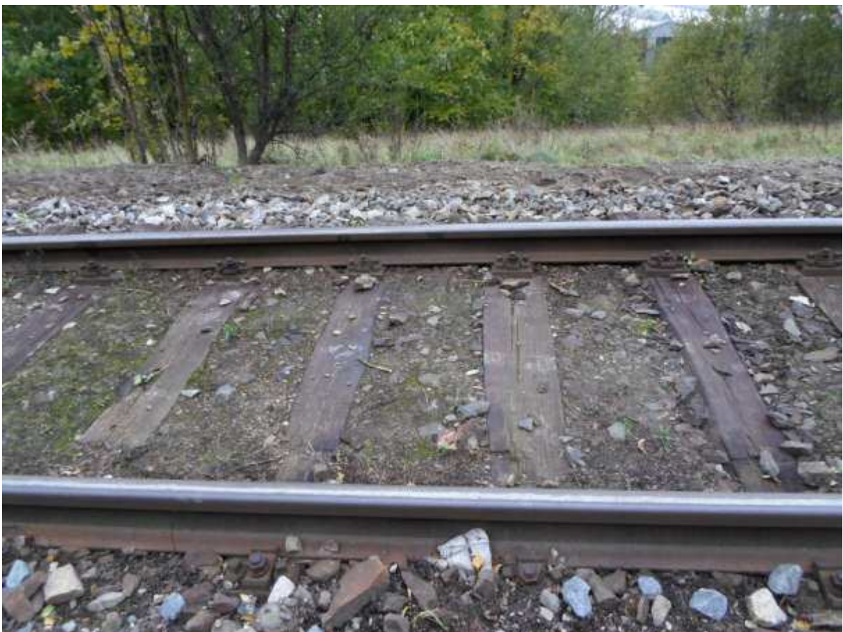
Obr. 10 Zanesené kolejové lože
