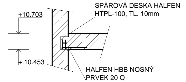
Uložení podesty do stěny
