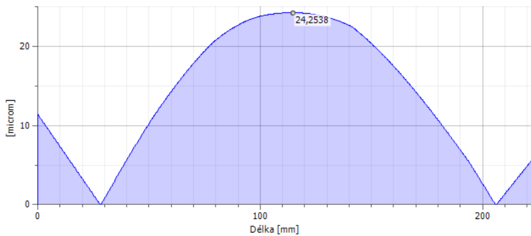
Výsledná superpozice průhybu předlokové hřídele pro směr otáčení 2
