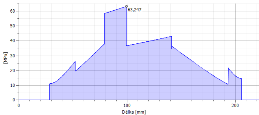
Průběh redukovaného napětí na předlokové hřídeli pro směr otáčení 1
