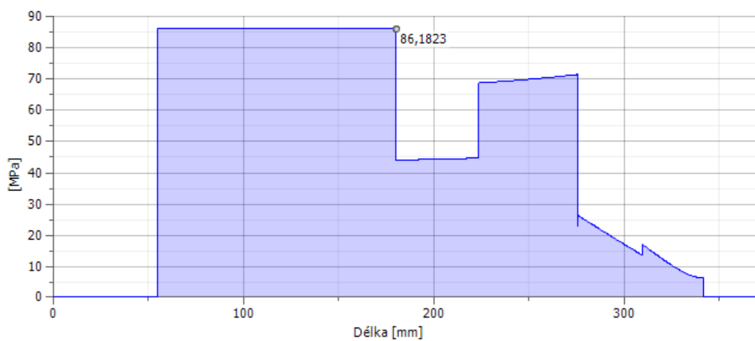
Průběh redukovaného napětí na výstupní hřídeli pro směr otáčení 2
