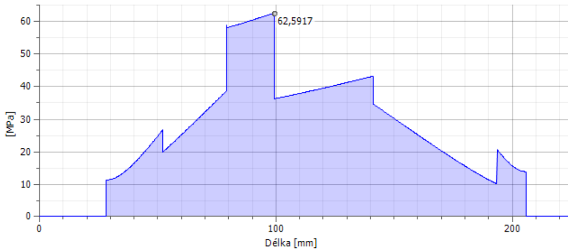
Průběh redukovaného napětí na předlokové hřídeli pro směr otáčení 2
