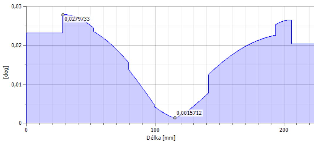
Výsledná superpozice natočení předlokové hřídele pro směr otáčení 1
