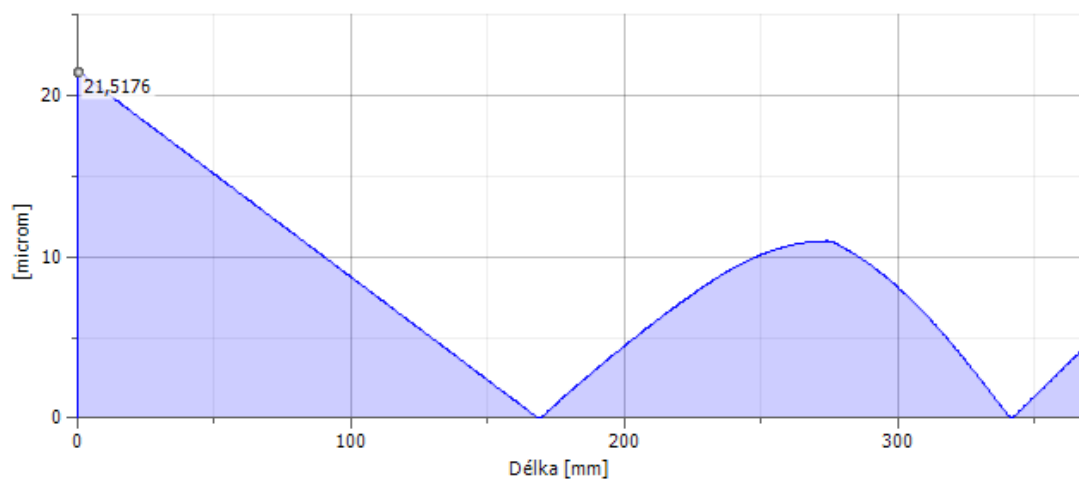
Výsledná superpozice průhybu výstupní hřídele pro směr otáčení 2
