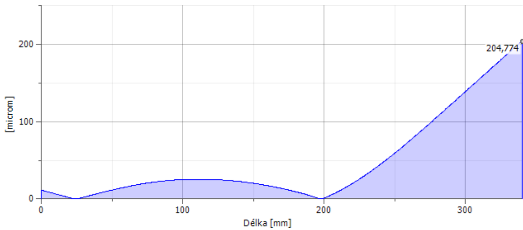
Výsledná superpozice průhybu vstupní hřídele pro směr otáčení 1
