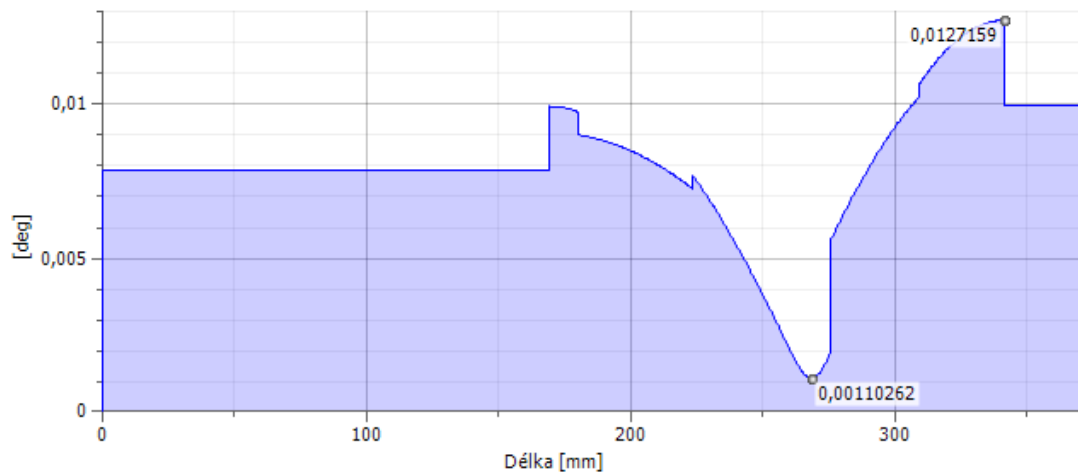
Výsledná superpozice natočení výstupní hřídele pro směr otáčení 1
