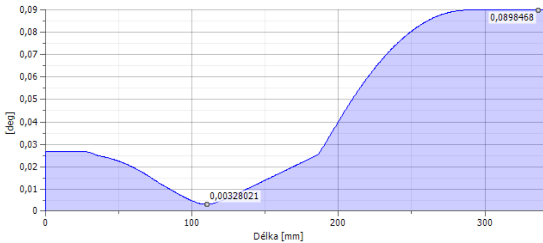
Výsledná superpozice natočení vstupní hřídele pro směr otáčení 2
