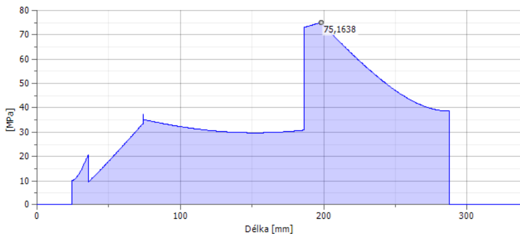
Průběh redukovaného napětí na vstupní hřídeli pro směr otáčení 2
