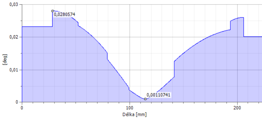
Výsledná superpozice natočení předlokové hřídele pro směr otáčení 2
