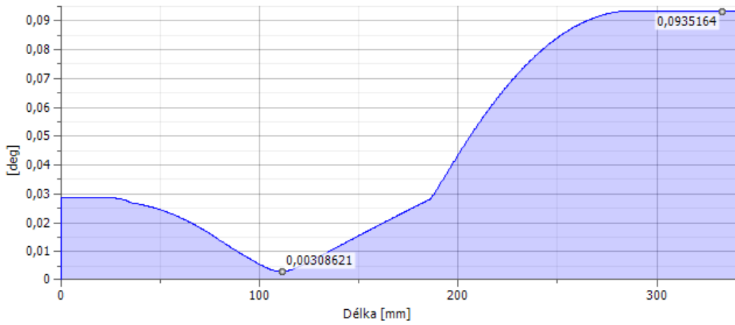
Výsledná superpozice natočení vstupní hřídele pro směr otáčení 1
