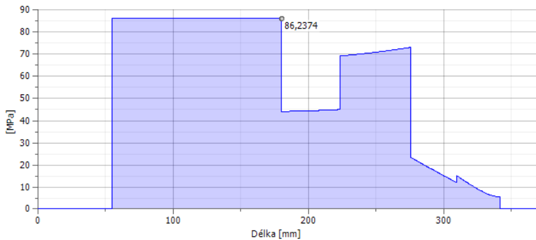
Průběh redukovaného napětí na výstupní hřídeli pro směr otáčení 1
