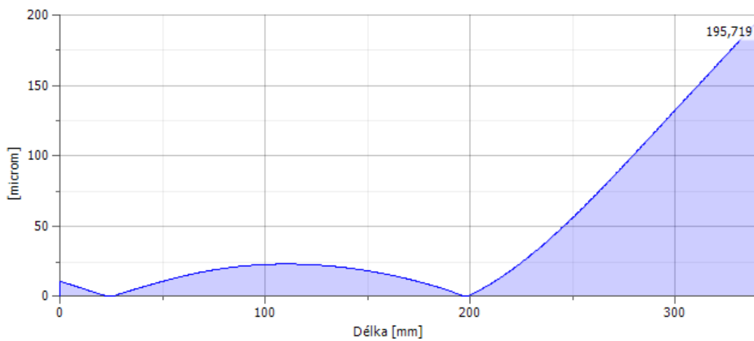
Výsledná superpozice průhybu vstupní hřídele pro směr otáčení 2
