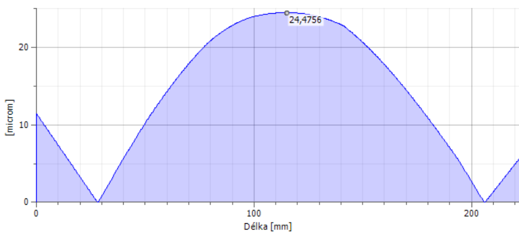
Výsledná superpozice průhybu předlokové hřídele pro směr otáčení 1
