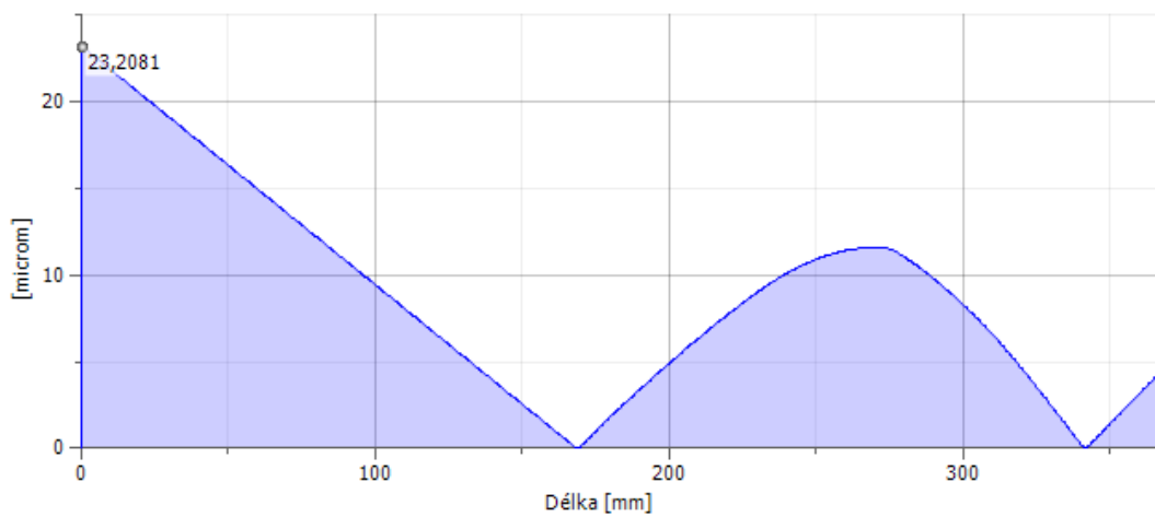
Výsledná superpozice průhybu výstupní hřídele pro směr otáčení 1
