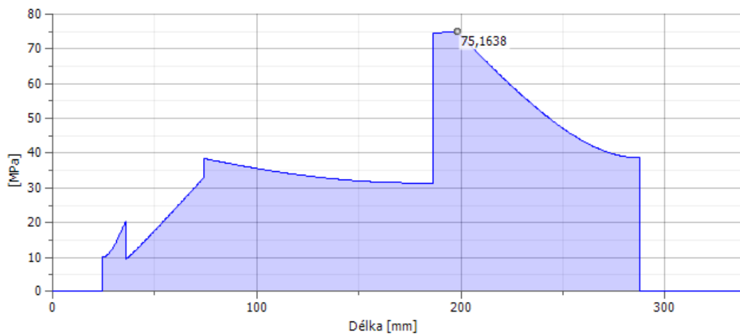
Průběh redukovaného napětí na vstupní hřídeli pro směr otáčení 1
