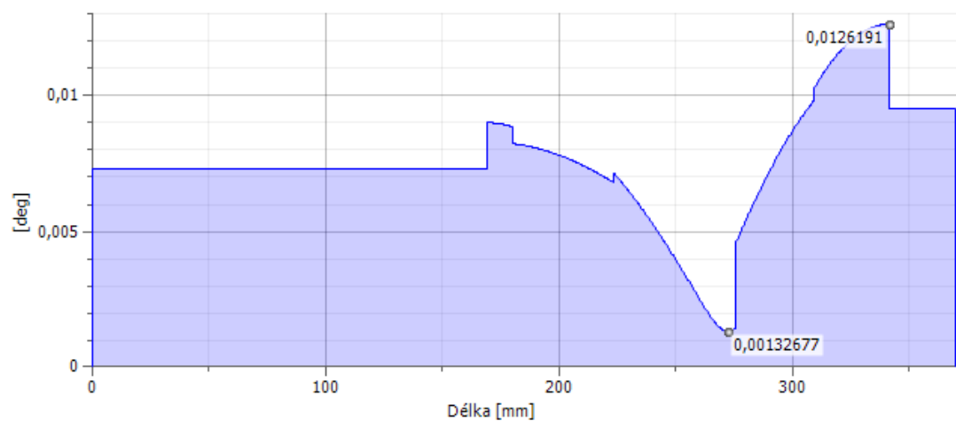
Výsledná superpozice natočení výstupní hřídele pro směr otáčení 2
