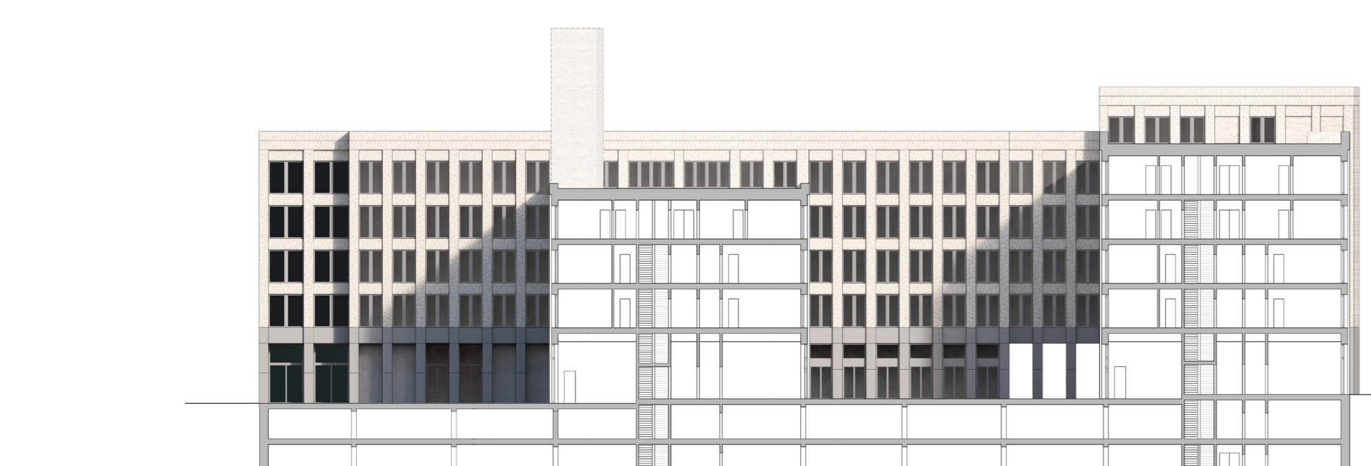
Rez vnitrobokem
