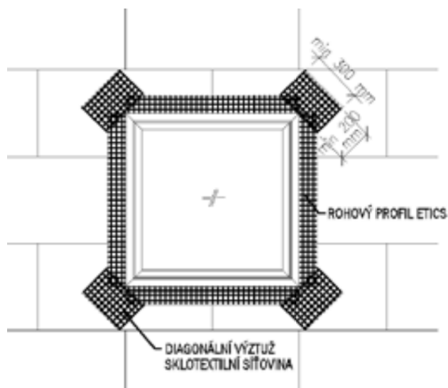
Obrázek 4: Detail vyztužení perlínkou u otvoru
