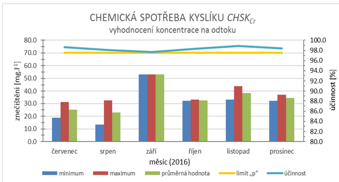
Graf č. 2 – Znečištění CHSK_{Cr} a účinnost čištění po rekonstrukci v roce 2016
