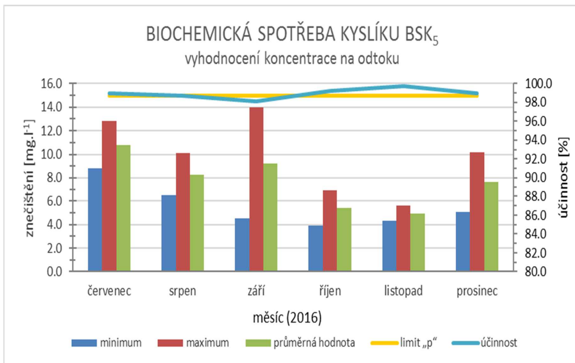
Graf č. 3 – Znečištění BSK 5 a účinnost čištění po rekonstrukci v roce 2016
