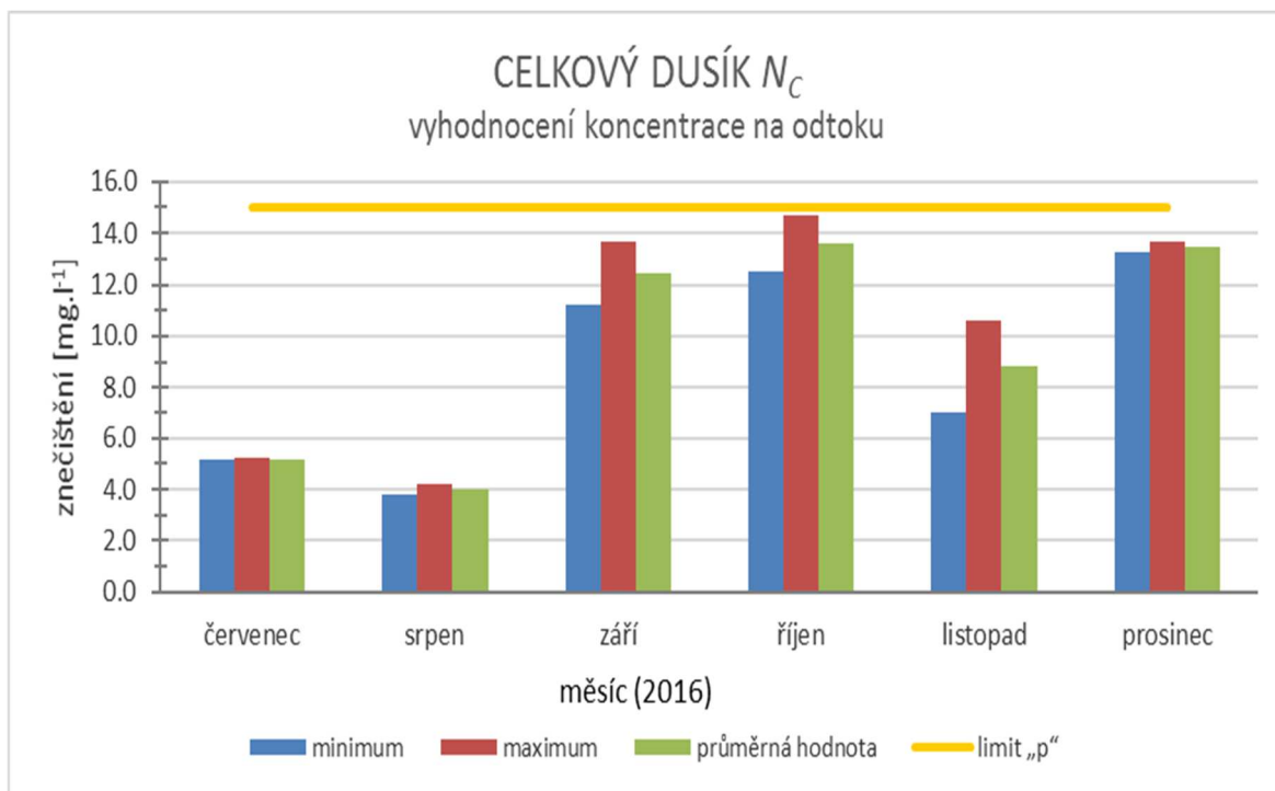
Graf č. 5 – Znečištění N_c po rekonstrukci v roce 2016
