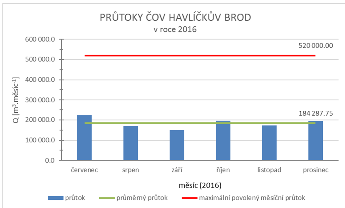
Graf č. 1 – Průtoky ČOV Havlíčkův Brod po rekonstrukci v roce 2016
