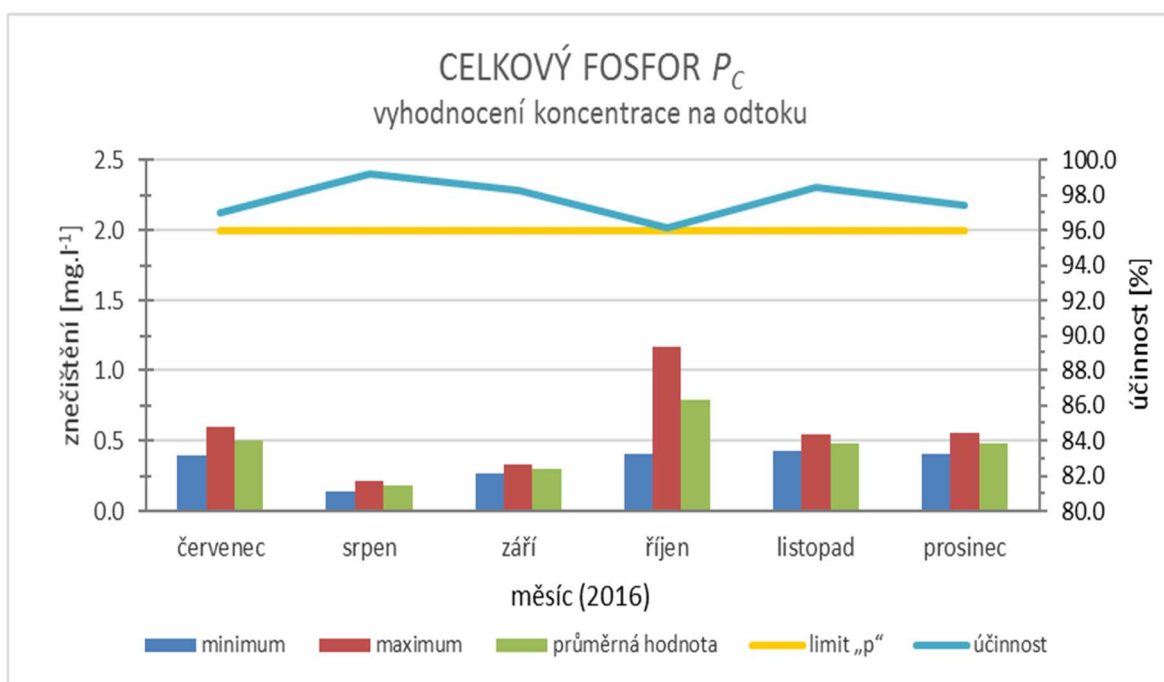
Graf č. 6 – Znečištění P_c a účinnost čištění po rekonstrukci v roce 2016
