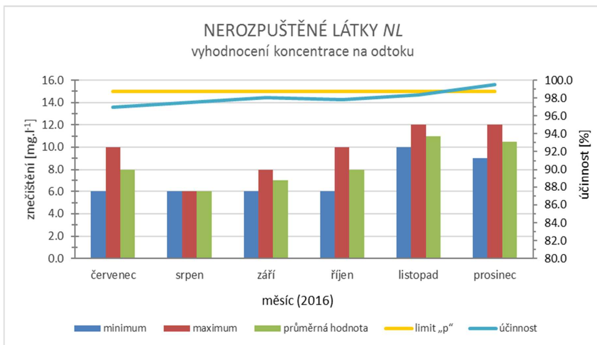
Graf č. 4 – Znečištění NL a účinnost čištění po rekonstrukci v roce 2016
