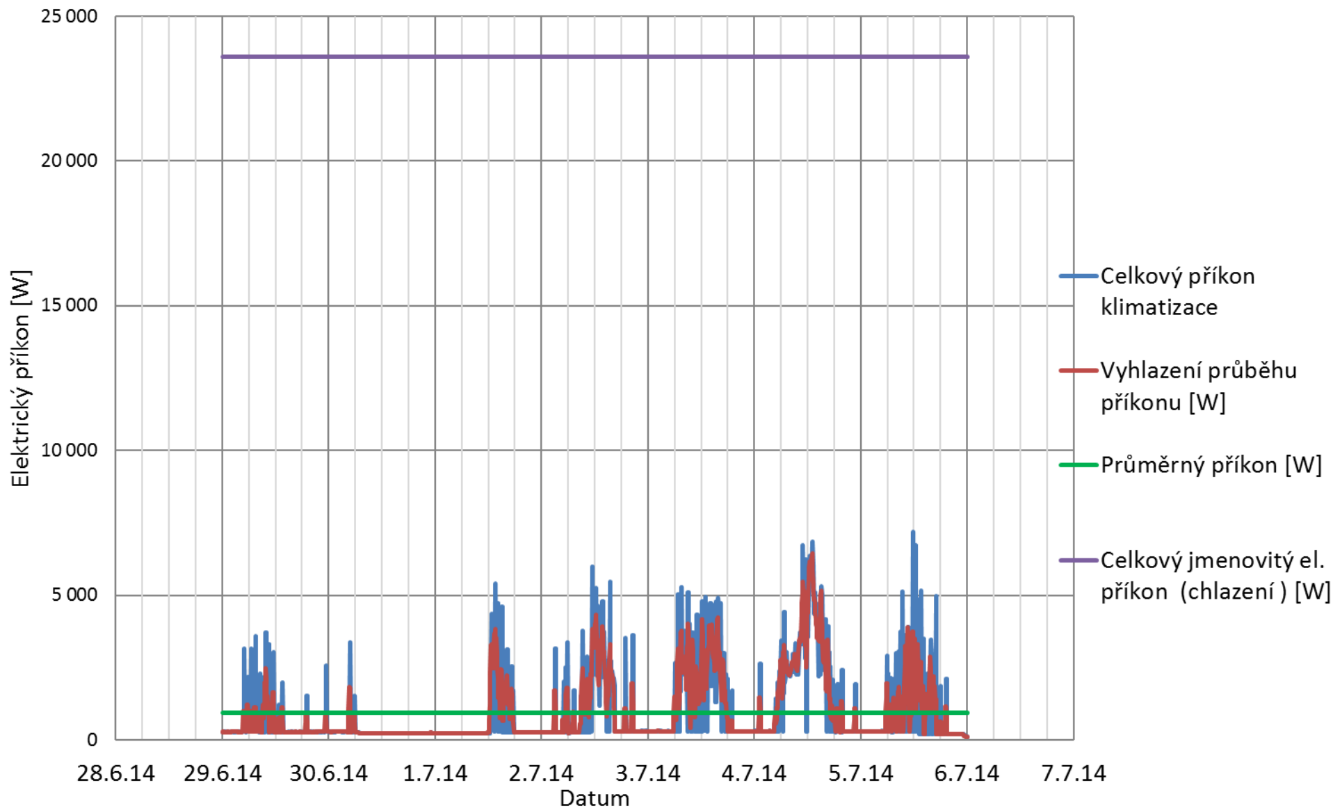
Celkový průběh elektrického příkonu klimatizačních zařízení pro 1.NP, 2.NP, 3.NP
