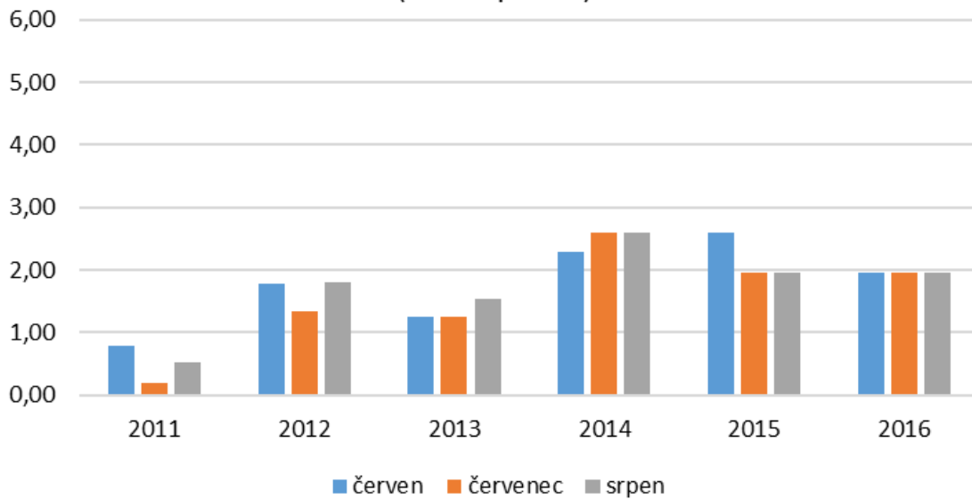
Měsíční měrné spotřeby pro letní období [kWh/m 2 ] (vnitřní plocha)
