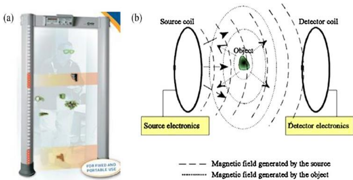
Obr. 4 WTMD – průchozí detektor kovů
