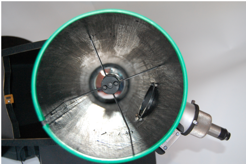
Obrázek : přichycení sek. zrcadla
