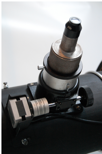
Obrázek : okulárový výtah
