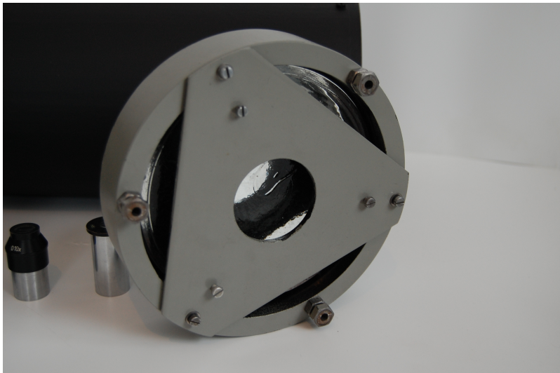
Obrázek : prim. zrcadlo na tubusu
