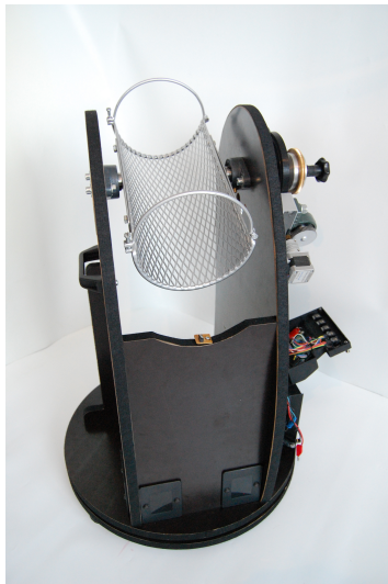
Obrázek : montáž odkrytovaná
