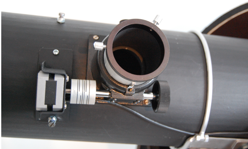
Obrázek : okulárový výtah
