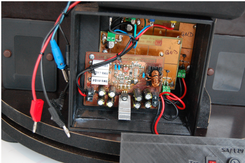
Obrázek : spínané zdroje
