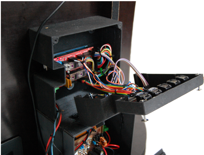
Obrázek : řídící jednotka
