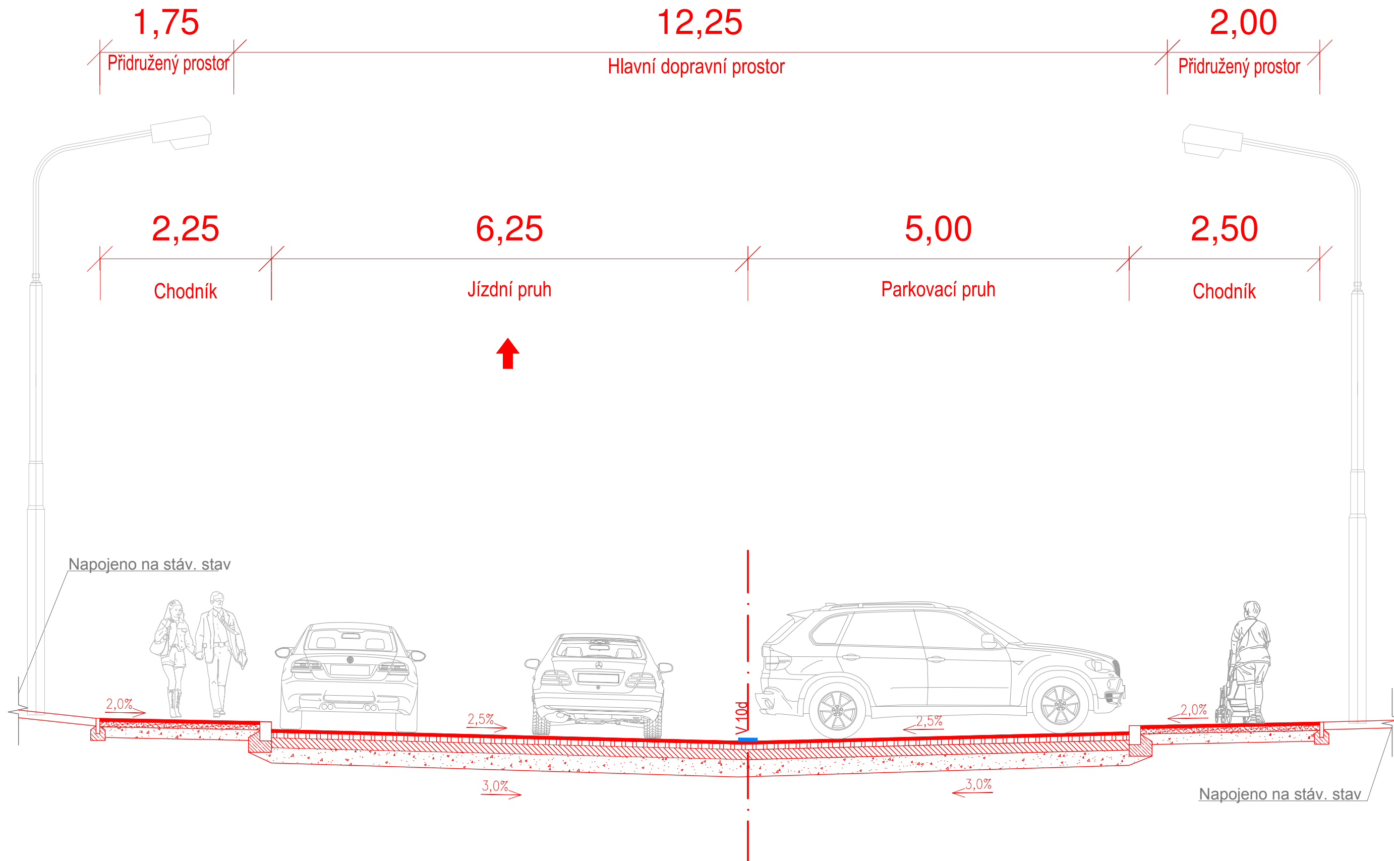
VZOROVÝ ŘEZ č. 4 ŘEZ V MÍSTĚ NOVÝCH KOLMÝCH PARKOVACÍCH STÁNÍ M = 1:50
