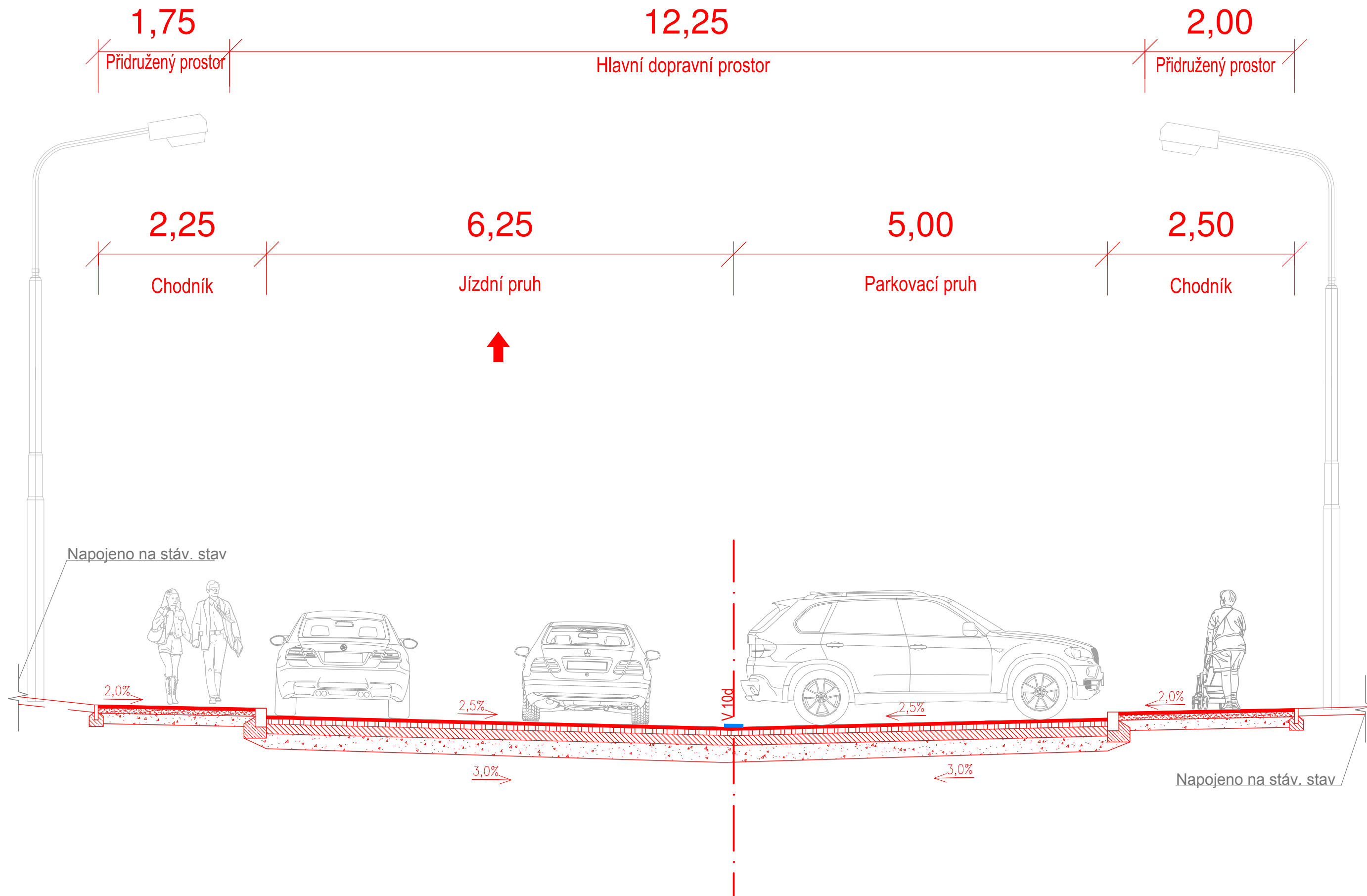
VZOROVÝ ŘEZ č. 4 ŘEZ V MÍSTĚ NOVÝCH KOLMÝCH PARKOVACÍCH STÁNÍ M = 1:50
