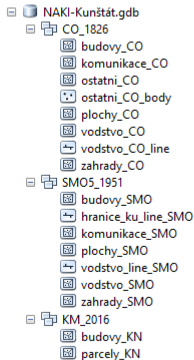
Obr. 9: Struktura geodatabáze při vektorizaci , zdroj: vlastní
