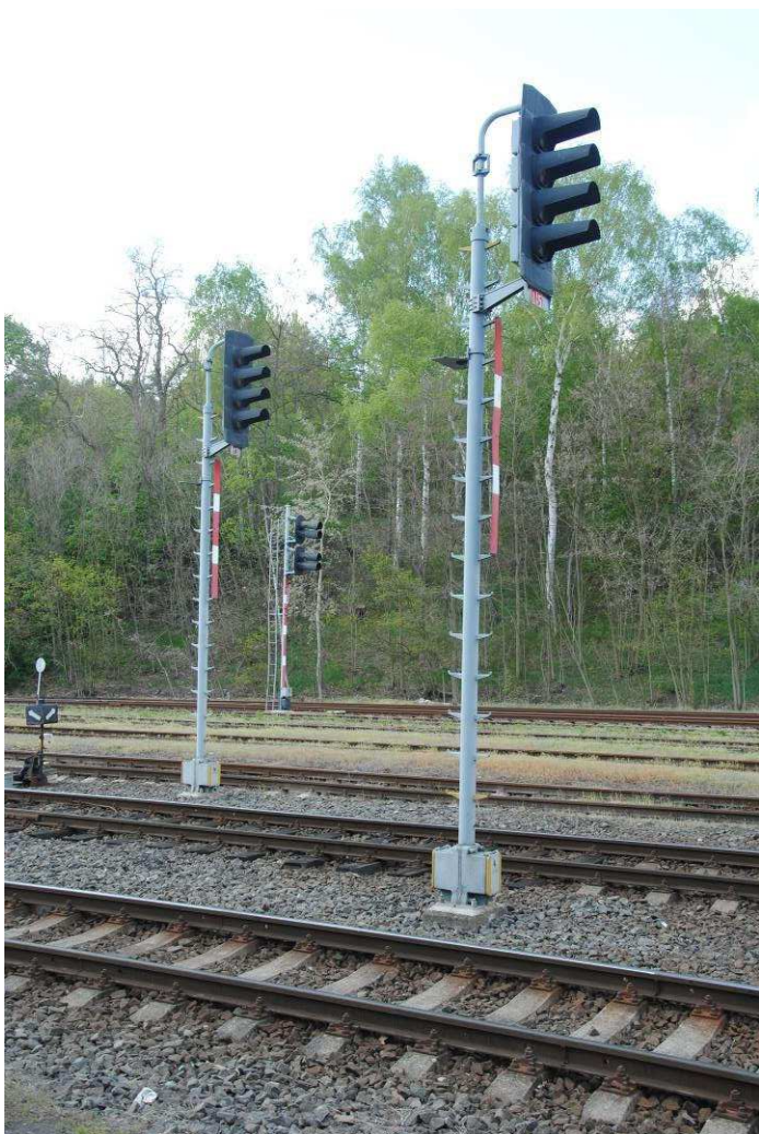
Obrázek 21: Odjezdová návěstidla dvojího typu – vzor AŽD 65 a AŽD 70
