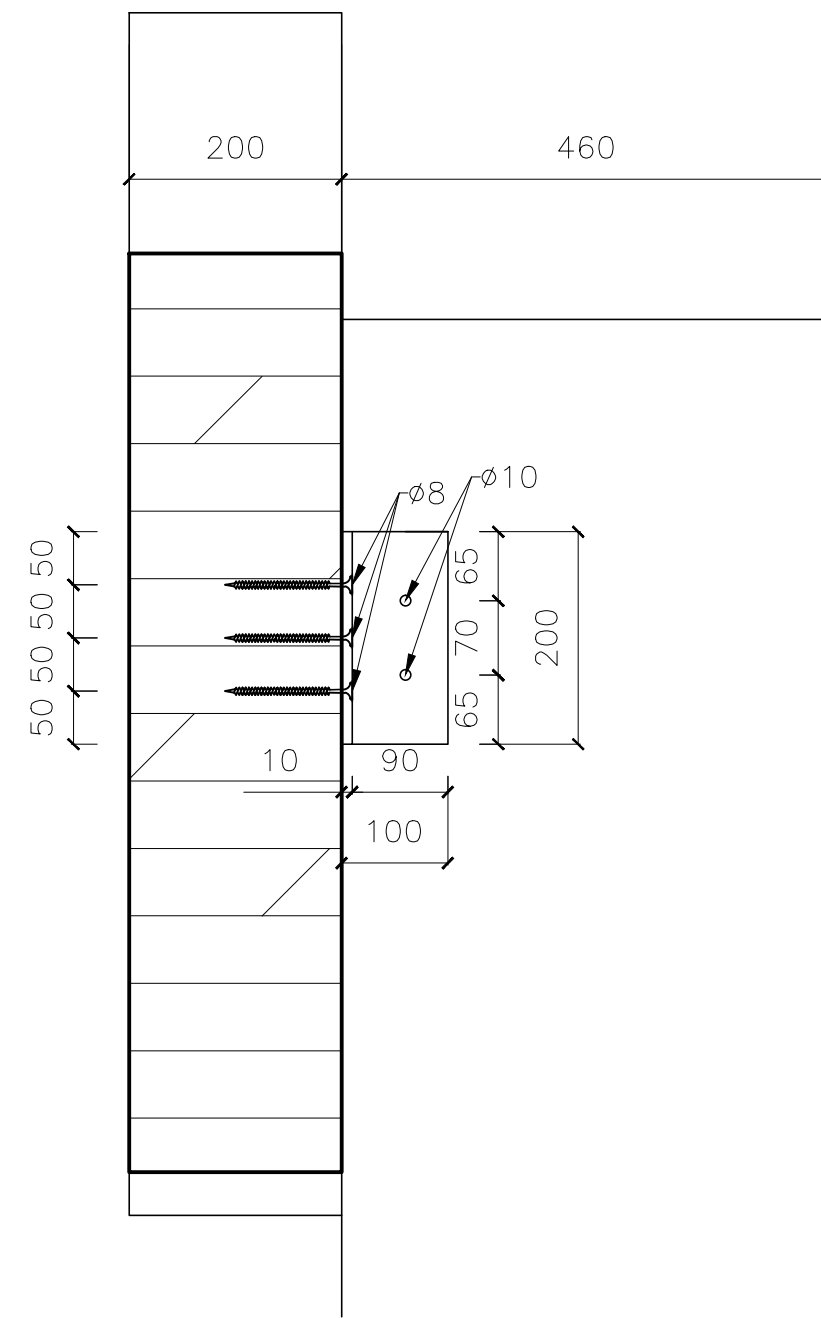
ŘEZ A - A'
