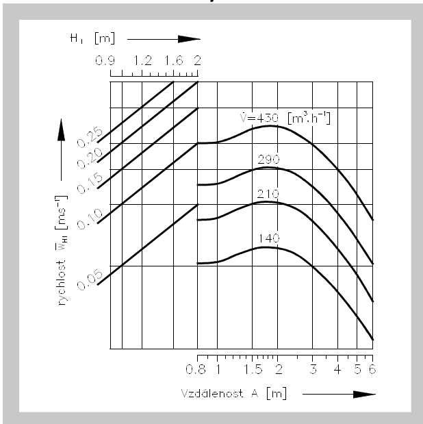
Diagram 9.3.3. Uspořádání vyústí jednořadé nebo víceřadé jestliže B \geq 4 m
