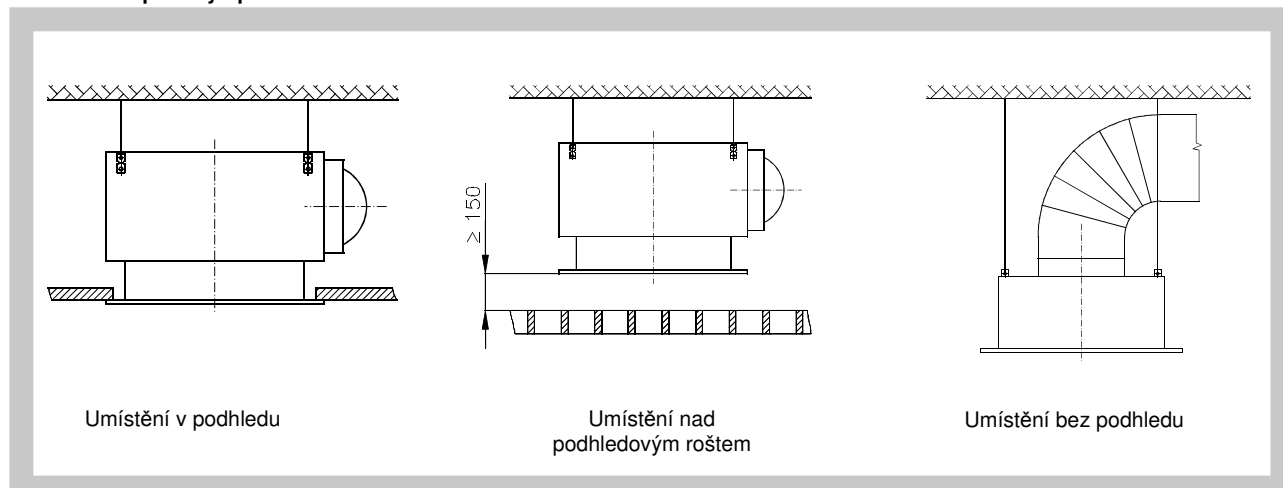
Obr. 11 Způsoby upevnění
