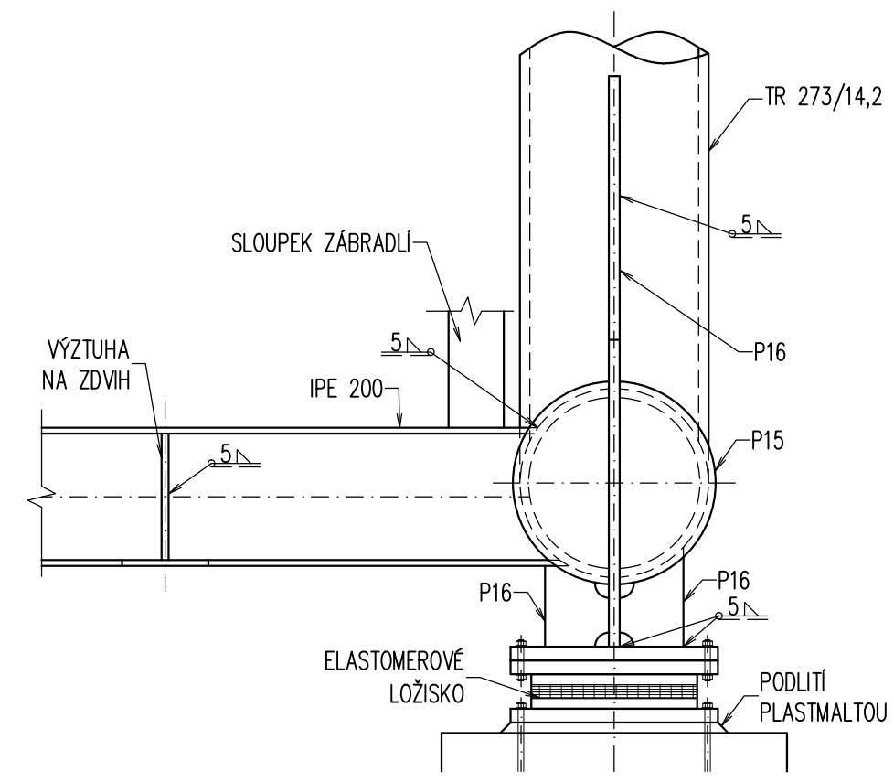
POHLED A 1:10
