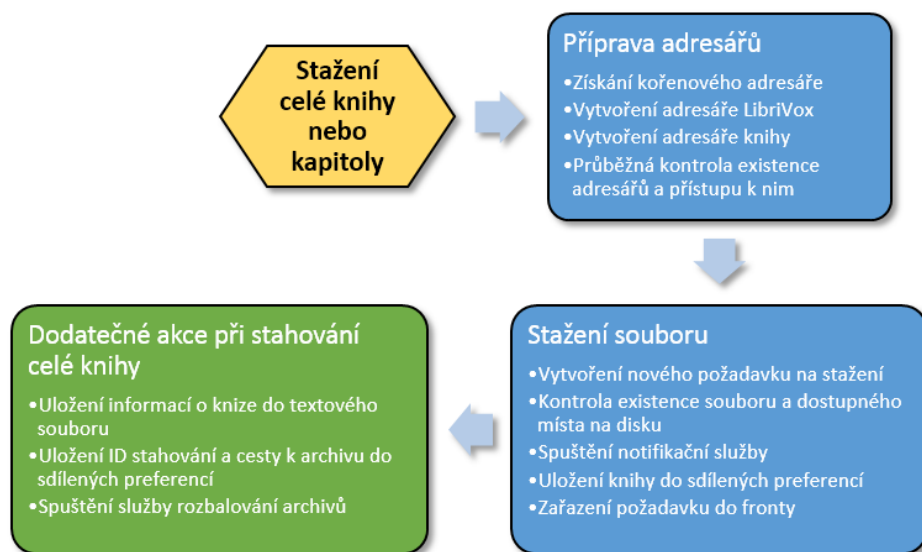
Obrázek 3.20: Proces stahování
