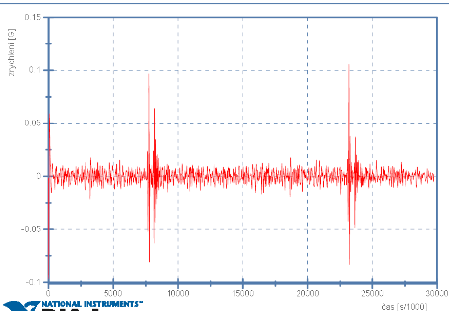
Škoda Octavia II - Přívěs se Škoda Rapid 20km/h - Senzor 2 - Boční zrychlení
