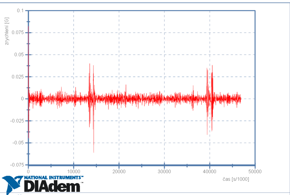
Škoda Octavia II - Zátěž v zavazadlovém prostoru 10km/h - Senzor 1 - Podélné zrychlení
