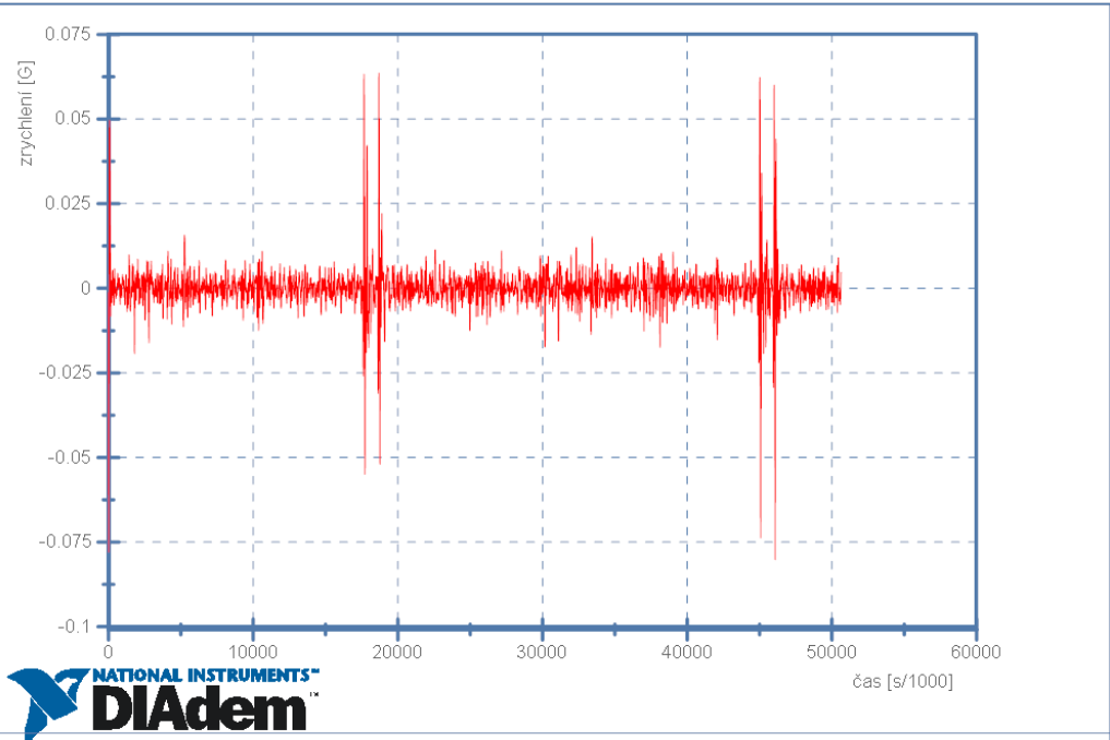
BMW 320d touring - 10km/h - Senzor 3 Podélné zrychlení
