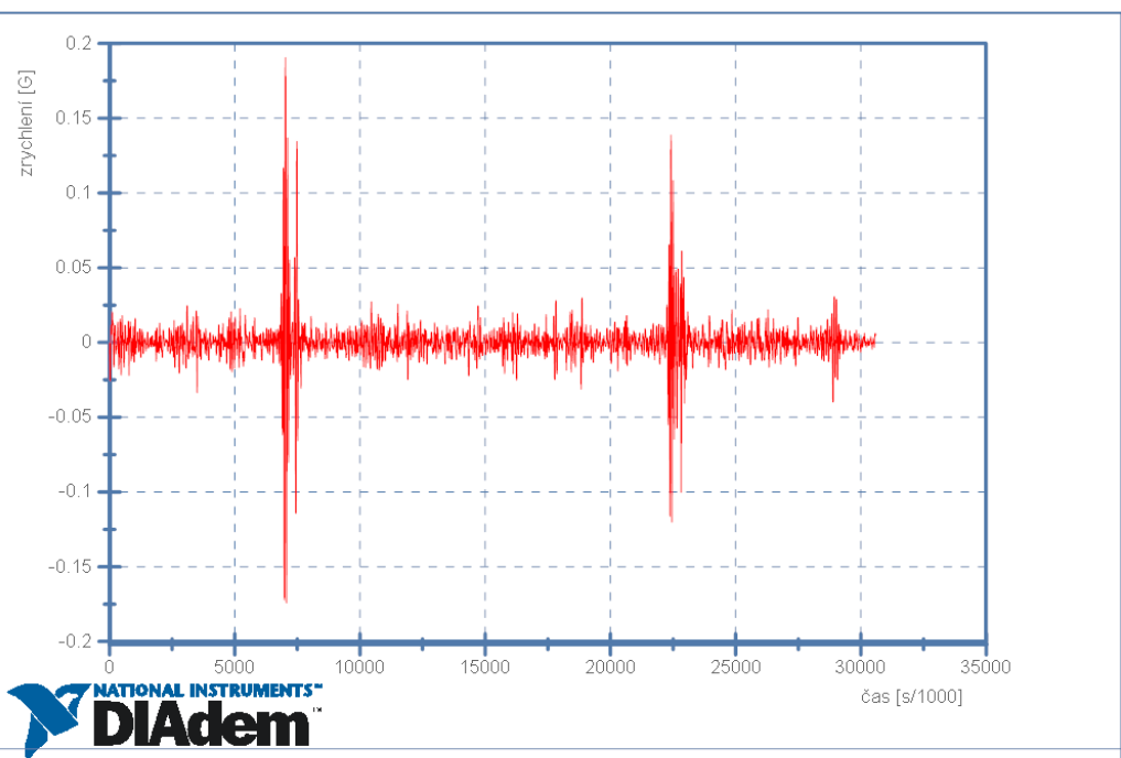
Škoda Rapid - 20km/h - Senzor 3 - Podélné zrychlení
