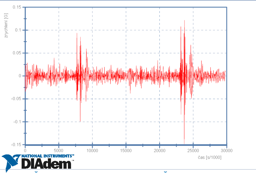
Škoda Octavia II - Přívěs se Škoda Rapid 20km/h - Senzor 2 - Podélné zrychlení
