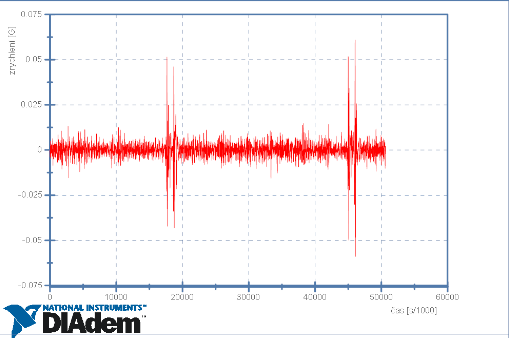
BMW 320d touring - 10km/h - Senzor 2 Podélné zrychlení
