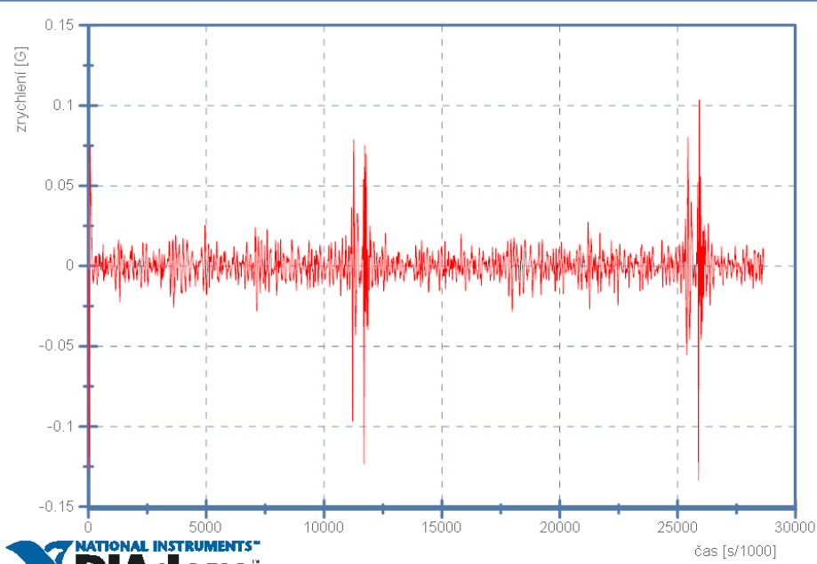
BMW 320d touring - 20km/h - Senzor 3 Boční zrychlení
