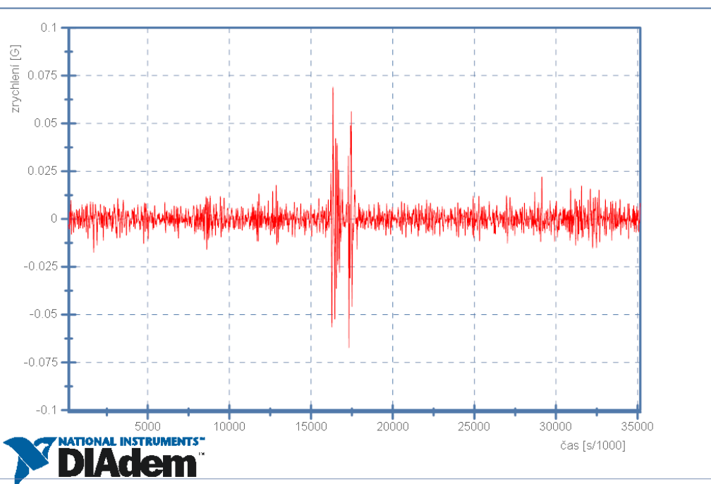
Škoda Rapid - 10km/h - Senzor 1 - Podélné zrychlení
