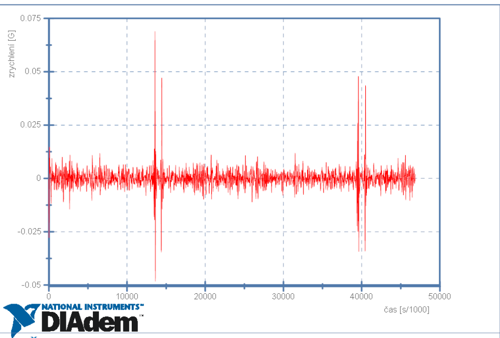
Škoda Octavia II - Zátěž v zavazadlovém prostoru 10km/h - Senzor 2 - Boční zrychlení
