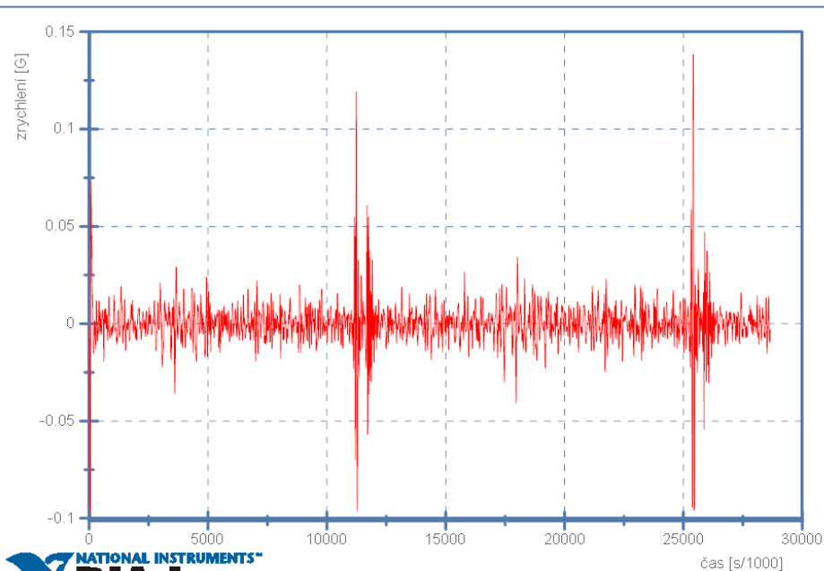
BMW 320d touring - 20km/h - Senzor 1 Podélné zrychlení
