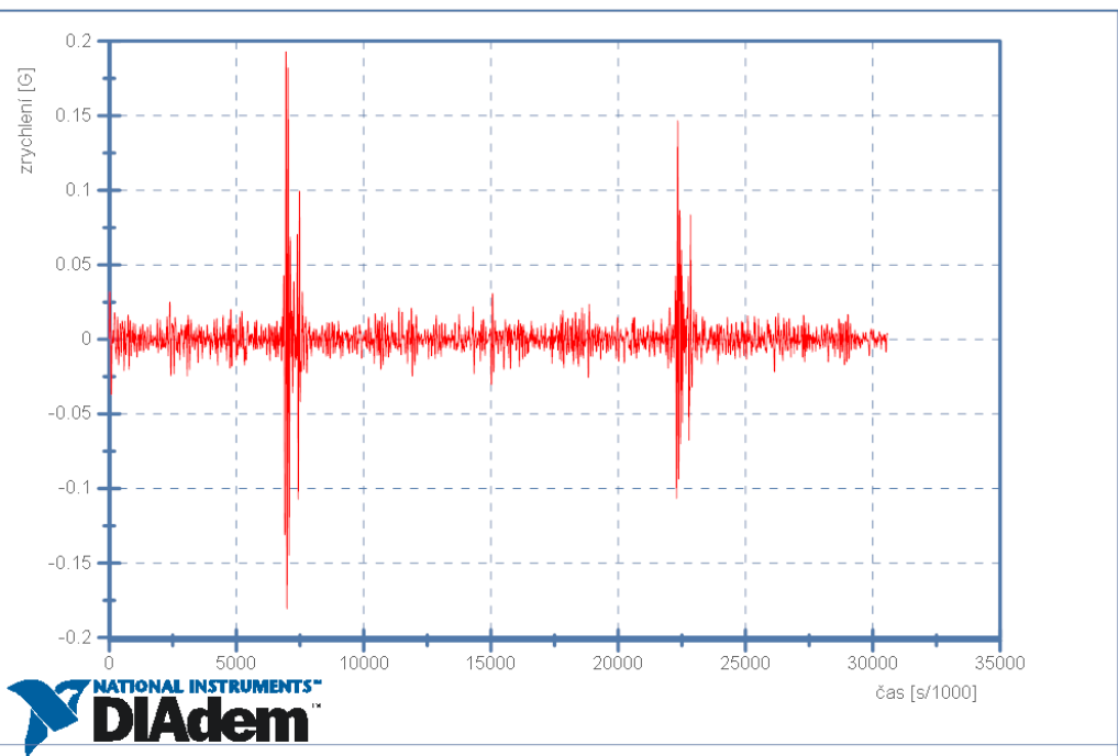
Škoda Rapid - 20km/h - Senzor 1 - Podélné zrychlení
