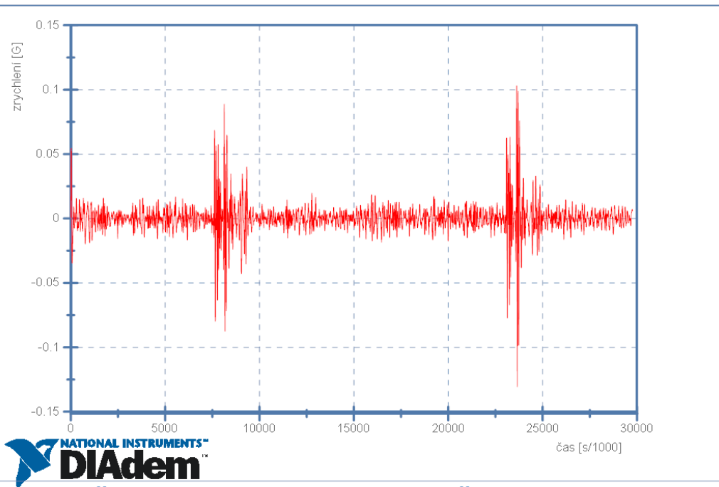
Škoda Octavia II - Přívěs se Škoda Rapid 20km/h - Senzor 3 - Podélné zrychlení
