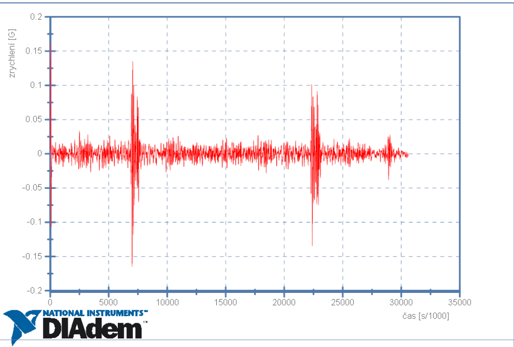
Škoda Rapid - 20km/h - Senzor 1 - Boční zrychlení
