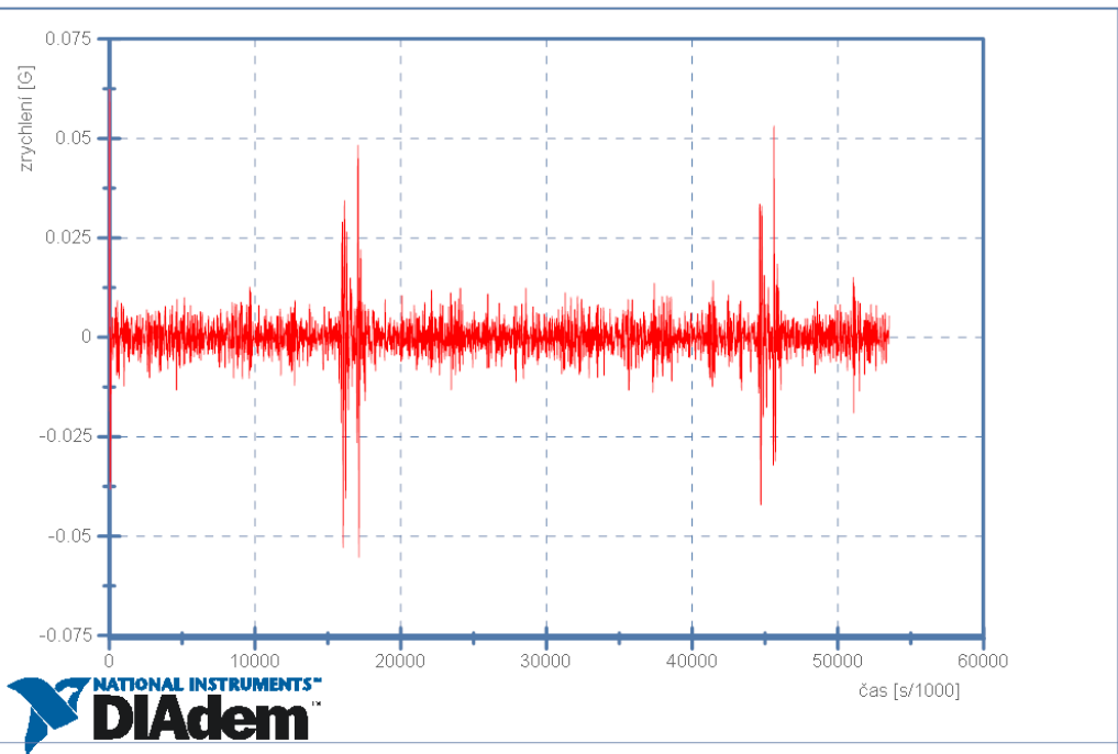
Škoda Octavia II - 10km/h - Senzor 1 - Podélné zrychlení
