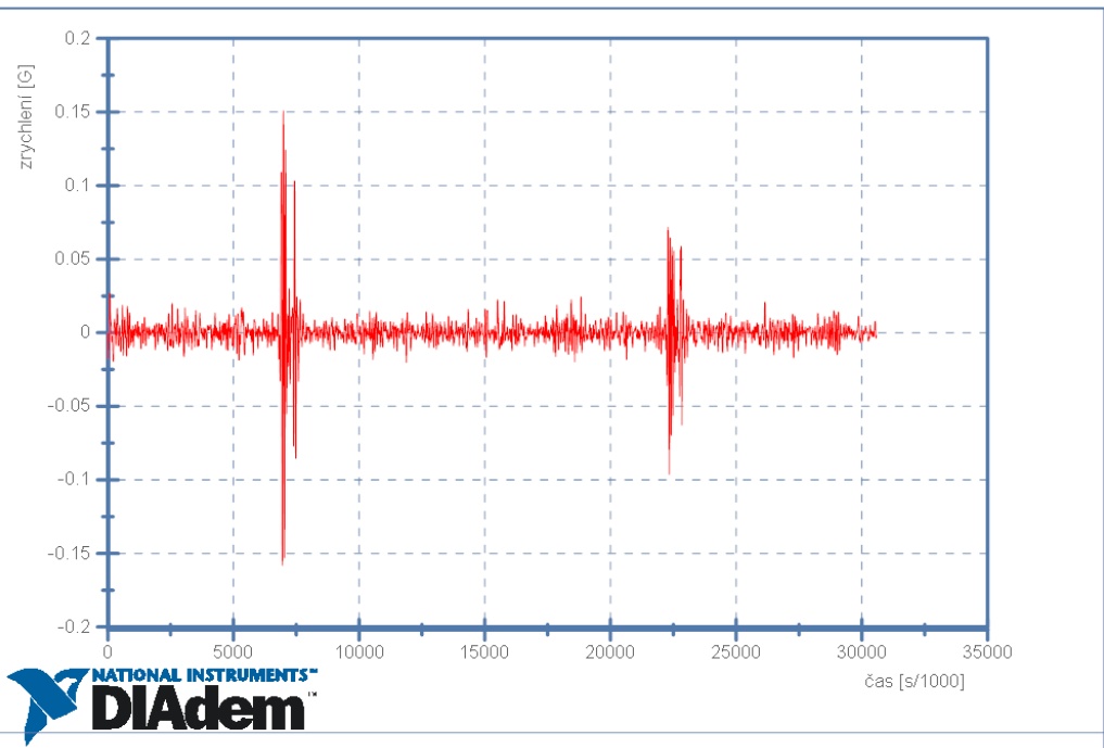
Škoda Rapid - 20km/h - Senzor 2 - Podélné zrychlení
