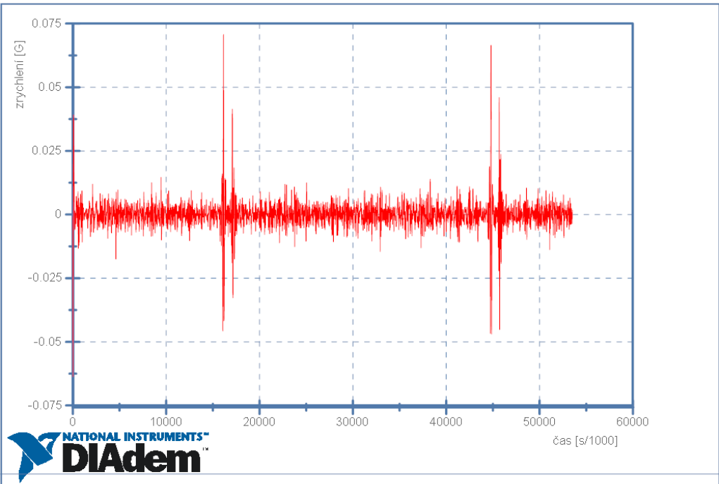
Škoda Octavia II - 10km/h - Senzor 2 - Podélné zrychlení
