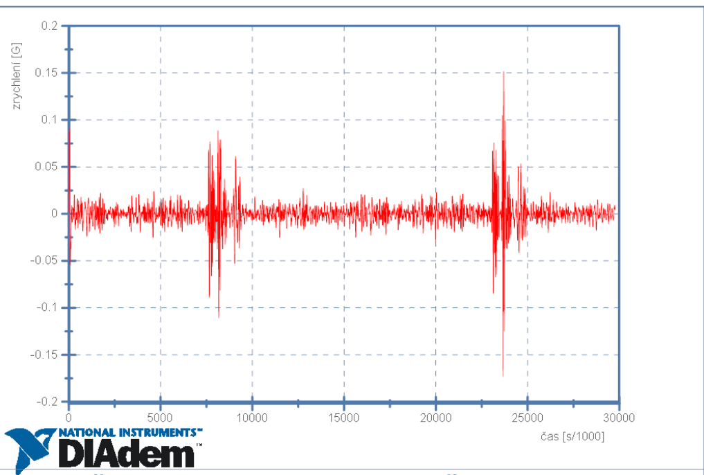
Škoda Octavia II - Přívěs se Škoda Rapid 20km/h - Senzor 1 - Podélné zrychlení
