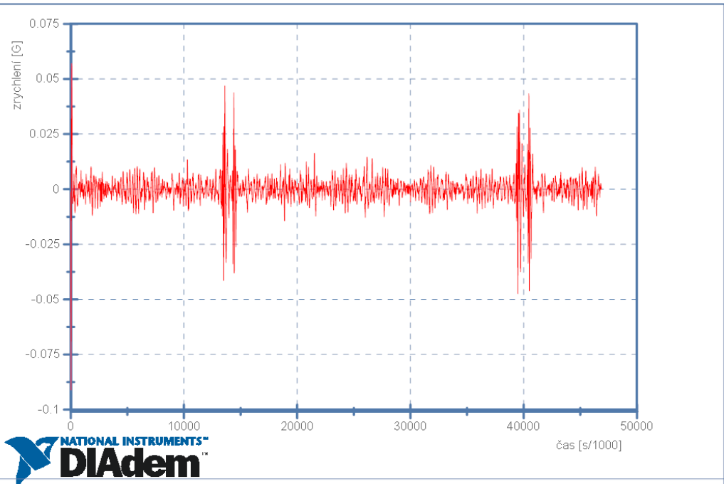
Škoda Octavia II - Zátěž v zavazadlovém prostoru 10km/h - Senzor 3 - Boční zrychlení
