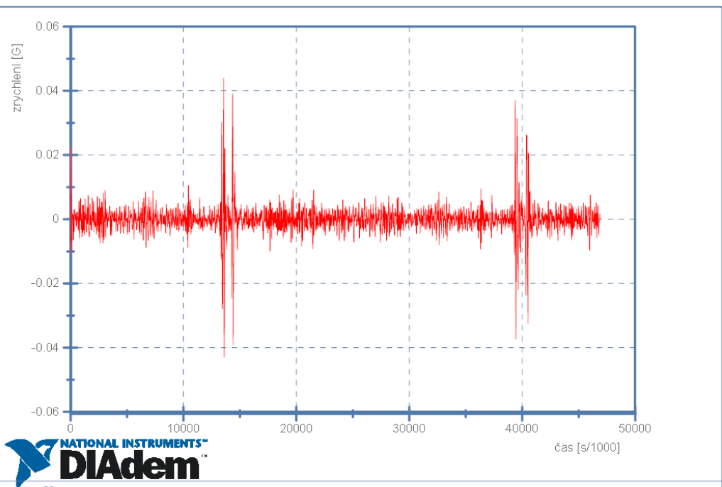
Škoda Octavia II - Zátěž v zavazadlovém prostoru 10km/h - Senzor 3 - Podélné zrychlení
