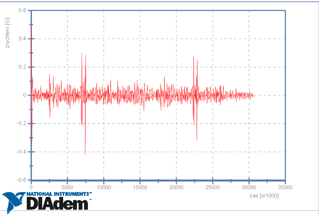
Škoda Rapid - 20km/h - Senzor 3 - Boční zrychlení
