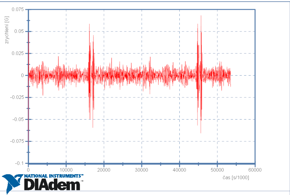
Škoda Octavia II - 10km/h - Senzor 3 - Boční zrychlení
