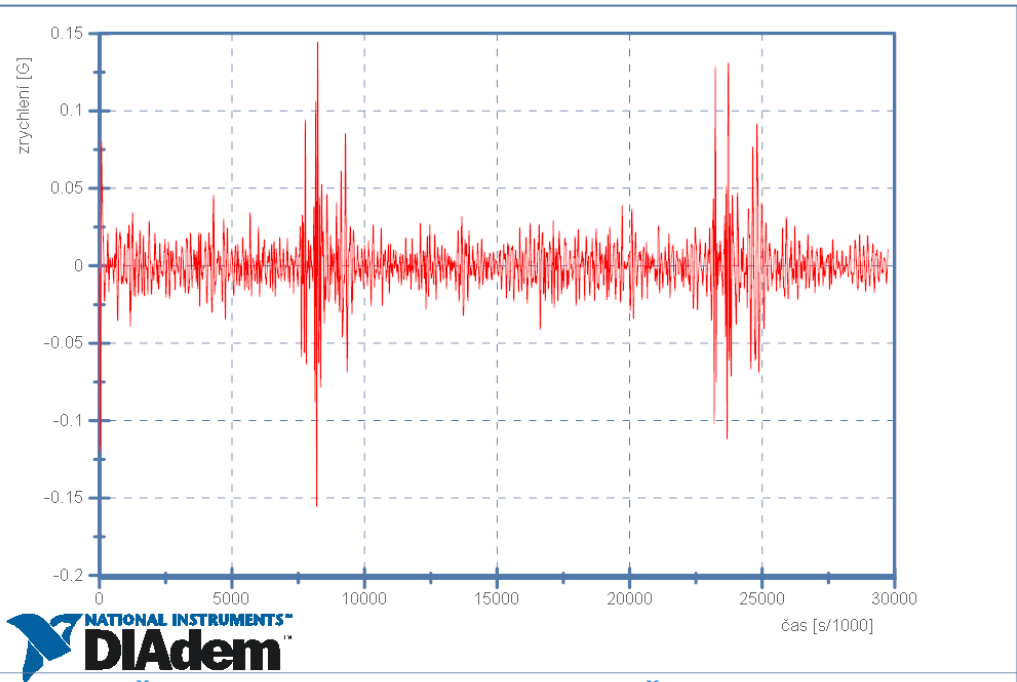
Škoda Octavia II - Přívěs se Škoda Rapid 20km/h - Senzor 3 - Boční zrychlení
