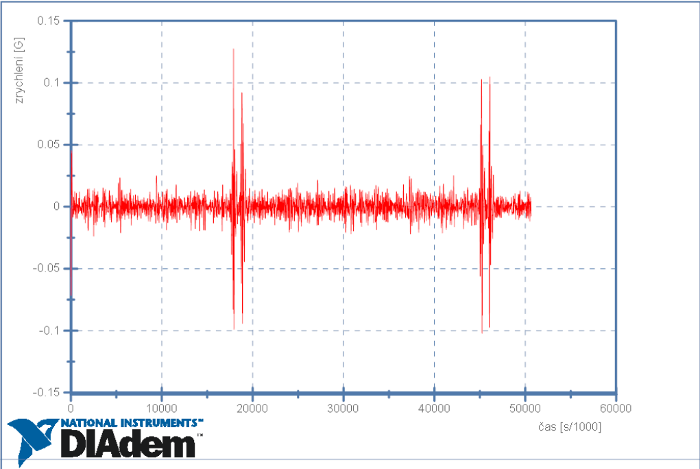
BMW 320d touring - 10km/h - Senzor 1 - Boční zrychlení
