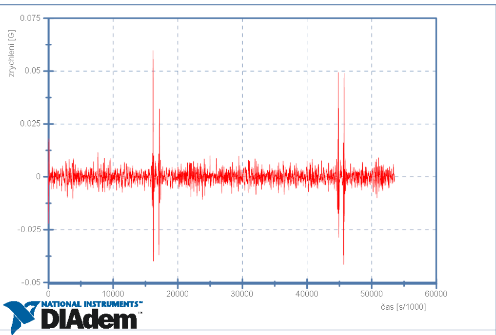
Škoda Octavia II - 10km/h - Senzor 2 - Boční zrychlení
