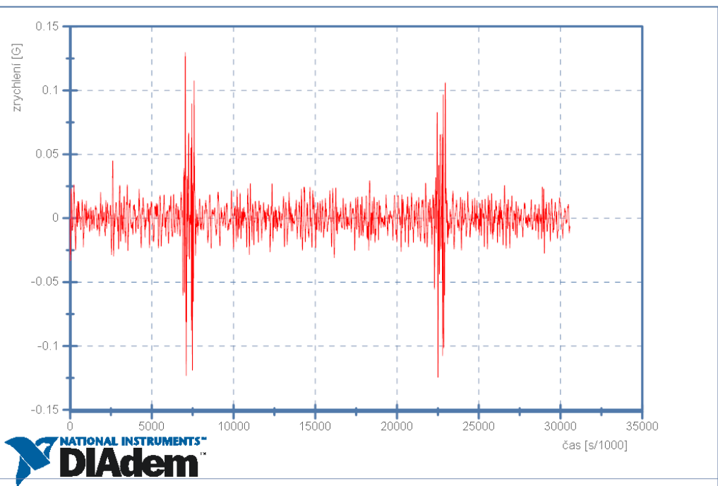
Škoda Rapid - 20km/h - Senzor 2 - Boční zrychlení
