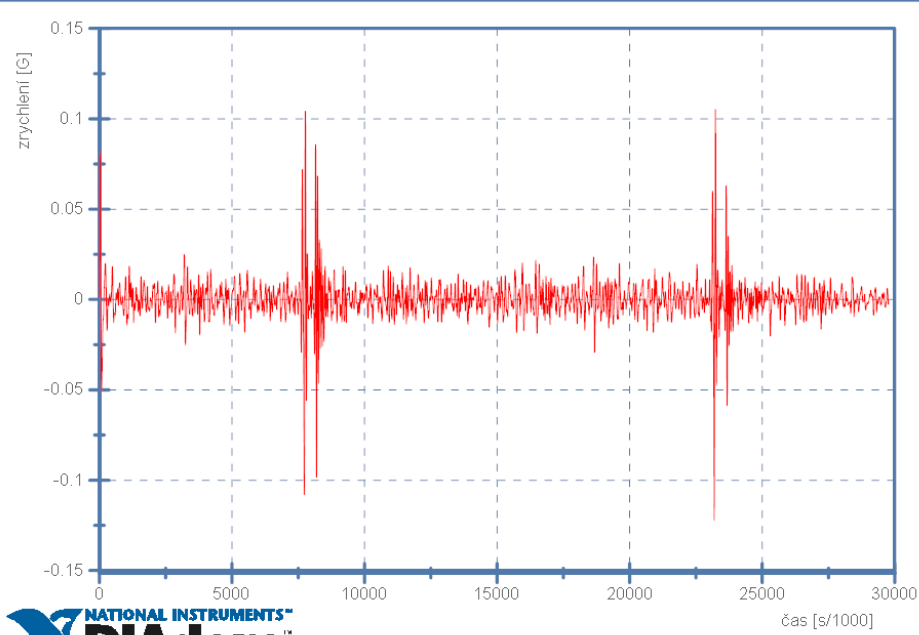
Škoda Octavia II - Přívěs se Škoda Rapid 20km/h - Senzor 1 - Boční zrychlení
