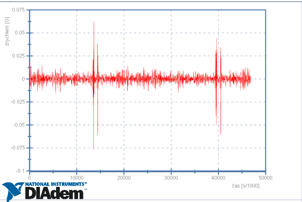
Škoda Octavia II - Zátěž v zavazadlovém prostoru 10km/h - Senzor 1 - Boční zrychlení
