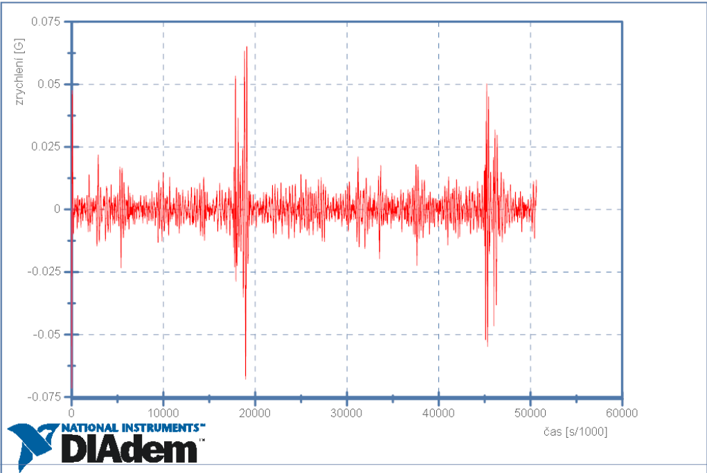
BMW 320d touring - 10km/h - Senzor 2 - Boční zrychlení
