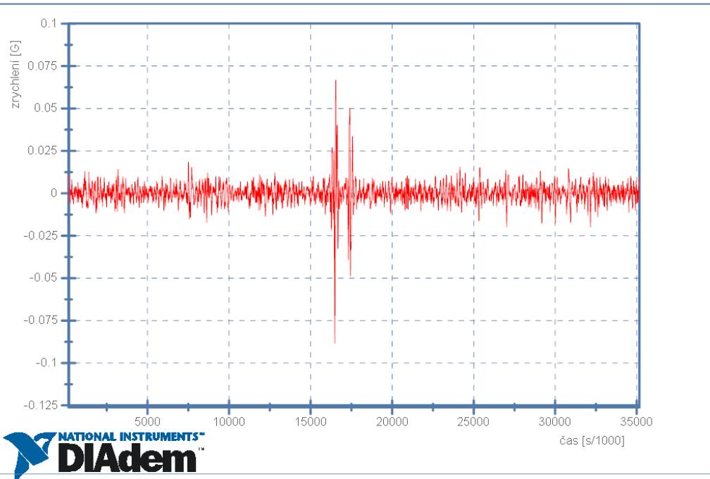
Škoda Rapid - 10km/h - Senzor 3 - Boční zrychlení
