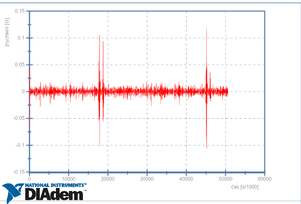
BMW 320d touring - 10km/h - Senzor 1 Podélné zrychlení
