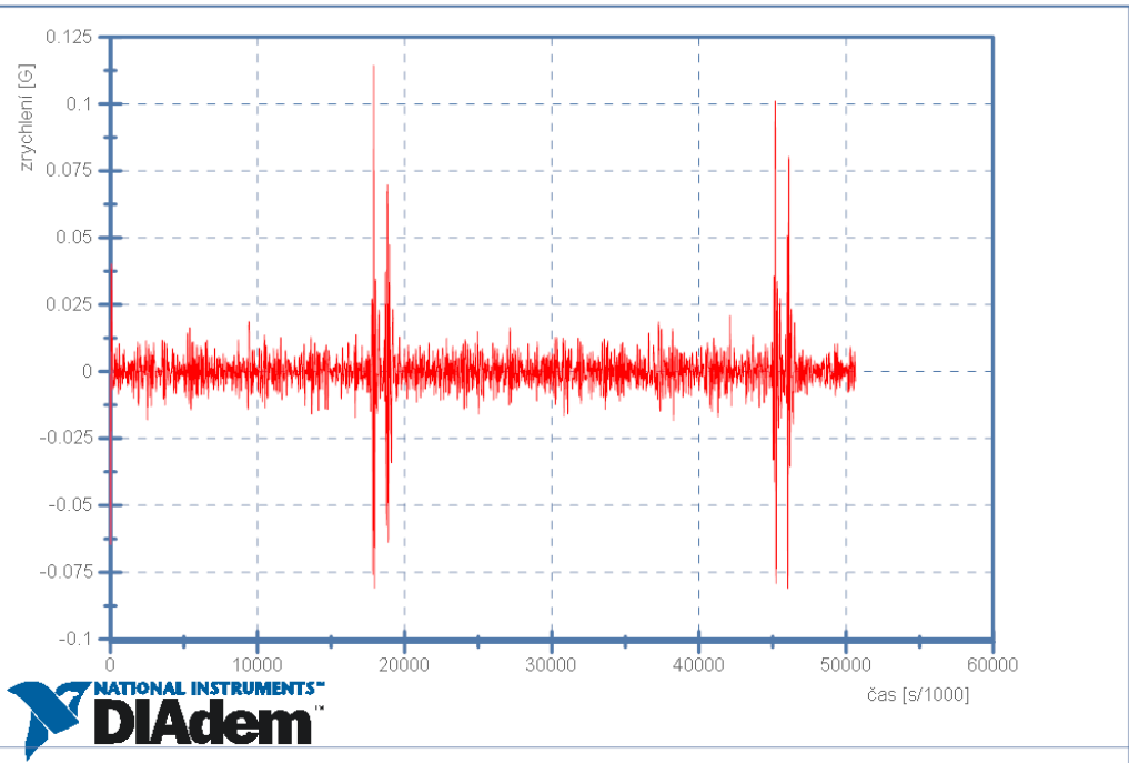
BMW 320d touring - 10km/h - Senzor 3 - Boční zrychlení
