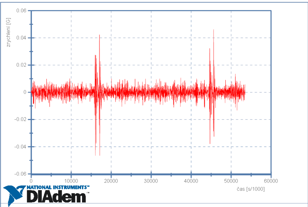
Škoda Octavia II - 10km/h - Senzor 3 - Podélné zrychlení
