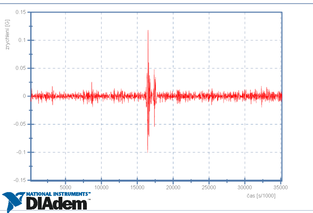
Škoda Rapid - 10km/h - Senzor 3 - Podélné zrychlení
