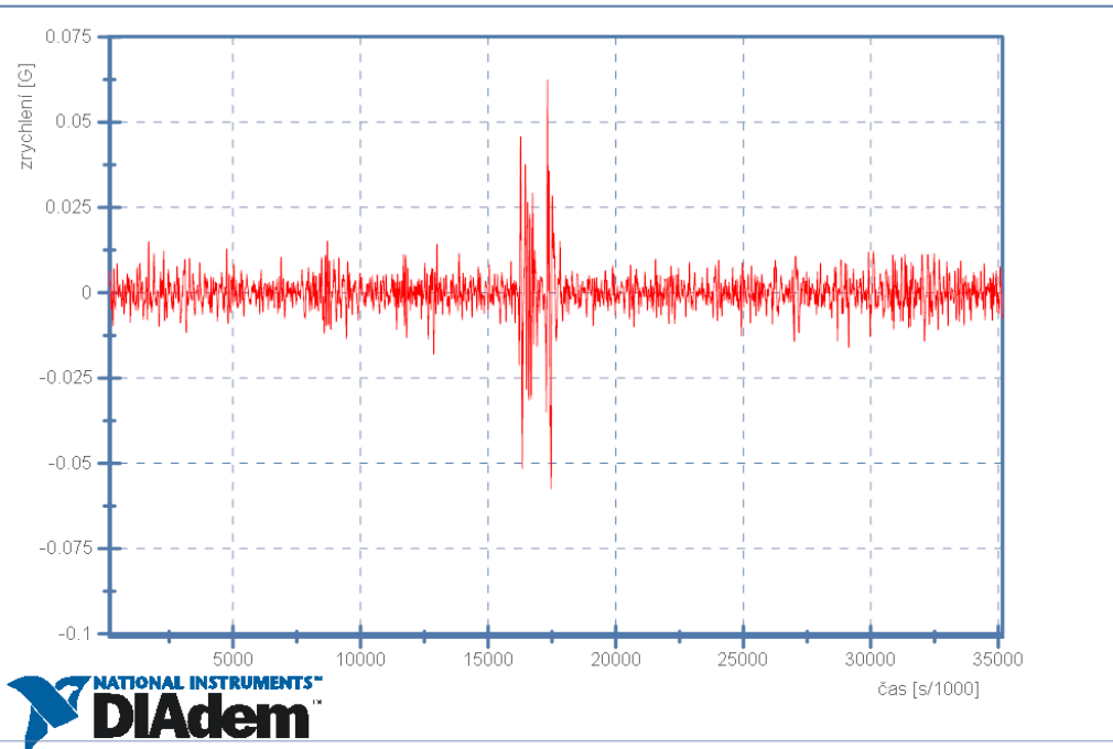
Škoda Rapid - 10km/h - Senzor 2 - Podélné zrychlení
