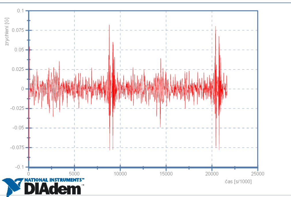
BMW 320d touring - 30km/h - Senzor 1 Podélné zrychlení
