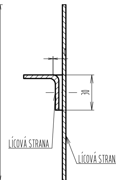
A-A (BEZ MĚŘITKA)
