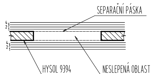
DETAIL C (BEZ MĚŘITKA)
