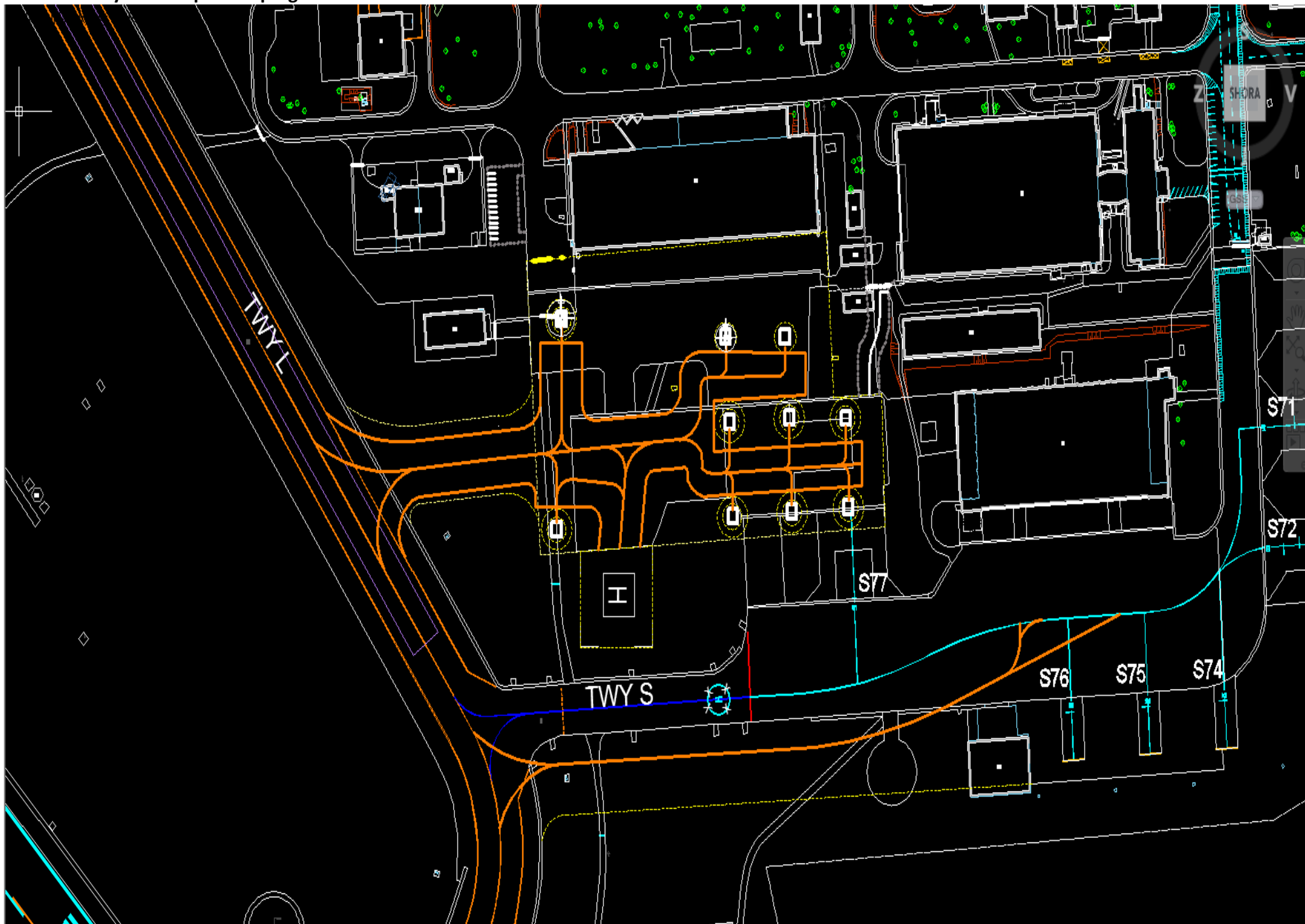
Příloha č. 1 Výkres heliportu v programu AutoCAD
