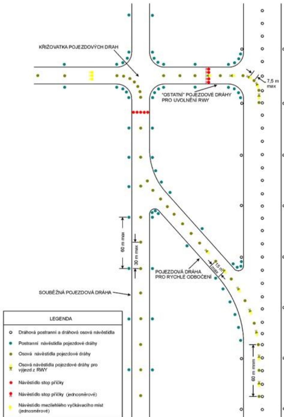
Obrázek 1.2 – Návěstidla TWY
