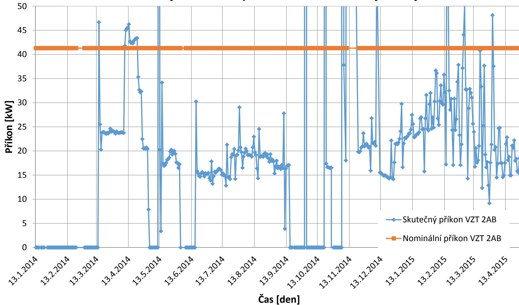
Obr. 8.16 – Skutečný a nominální příkon vzduchotechnické jednotky 2AB
