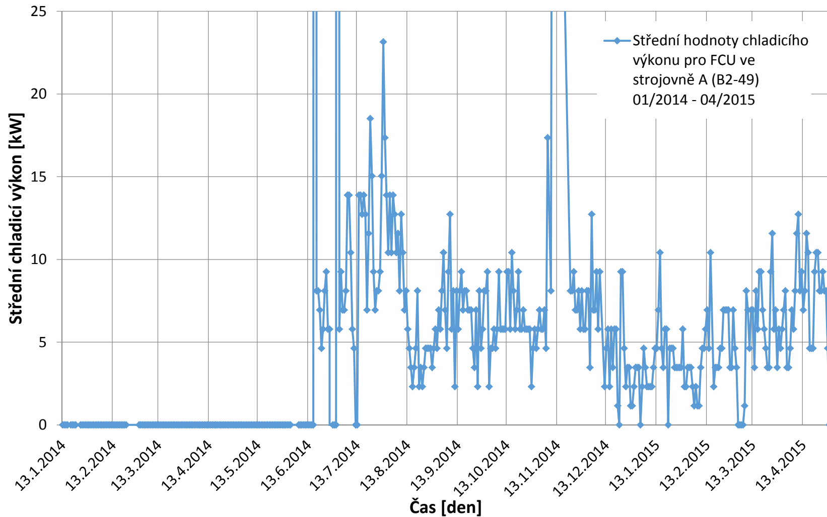
Obr. 8.1 – Střední hodnoty chladicího výkonu pro FCU ve strojovně A (B2-49)
