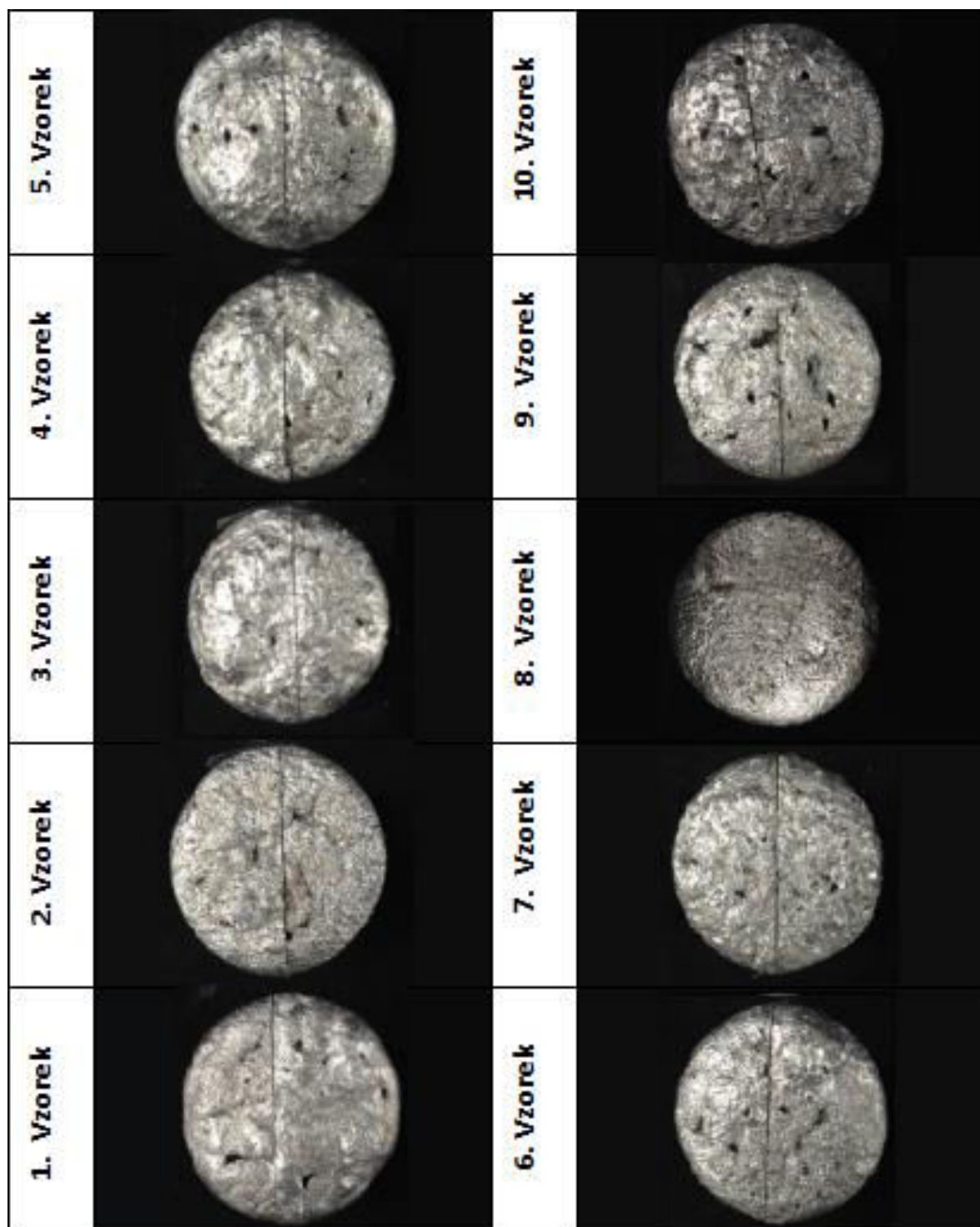
Příloha č. 5 Povrchy vzorků ze slitiny ENAC-43100 z materiálu o složení 100 % housky, 0 % vrat
