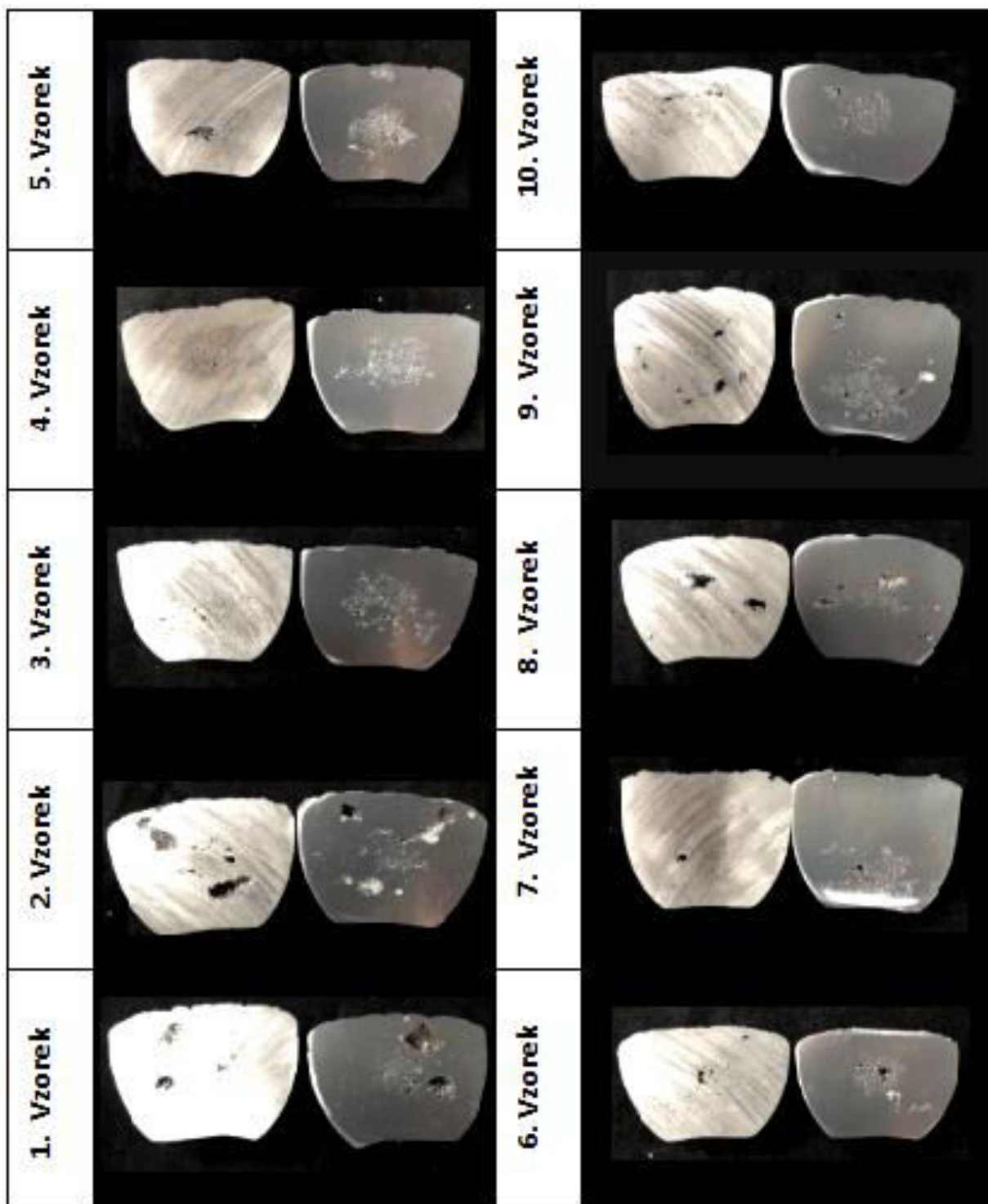
Příloha č. 2 Řezy vzorků ze slitiny ENAC-43.100 z materiálu o složení 60 % housky, 40 % vrat
