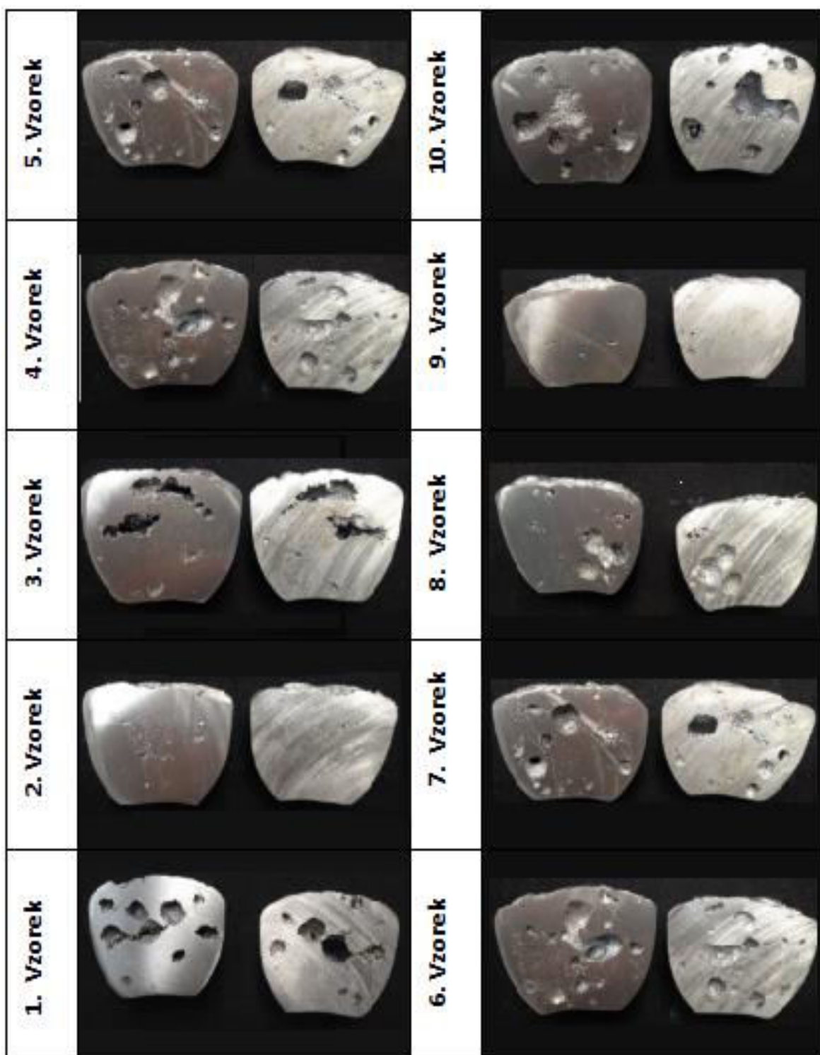
Příloha č. 6 Řezy vzorků ze slitiny EN AC-43 100 z materiálu o složení 100 % housky, 0 % vrat
