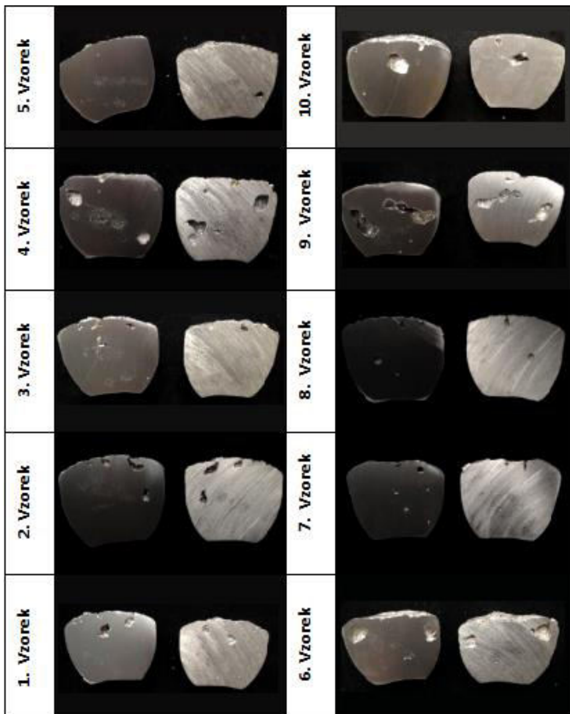
Příloha č. 4 Řezy vzorků ze slitiny EN AC-42 100 z materiálu o složení 60 % housky, 40 % vrat
