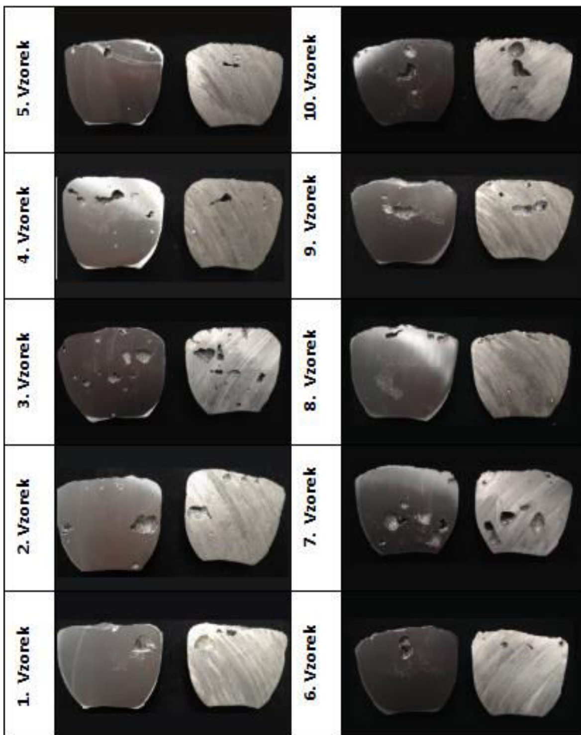
Příloha č. 8 Řezy vzorků ze slitiny EN AC-42 100 z materiálu o složení 100 % housky, 0 % vrat
