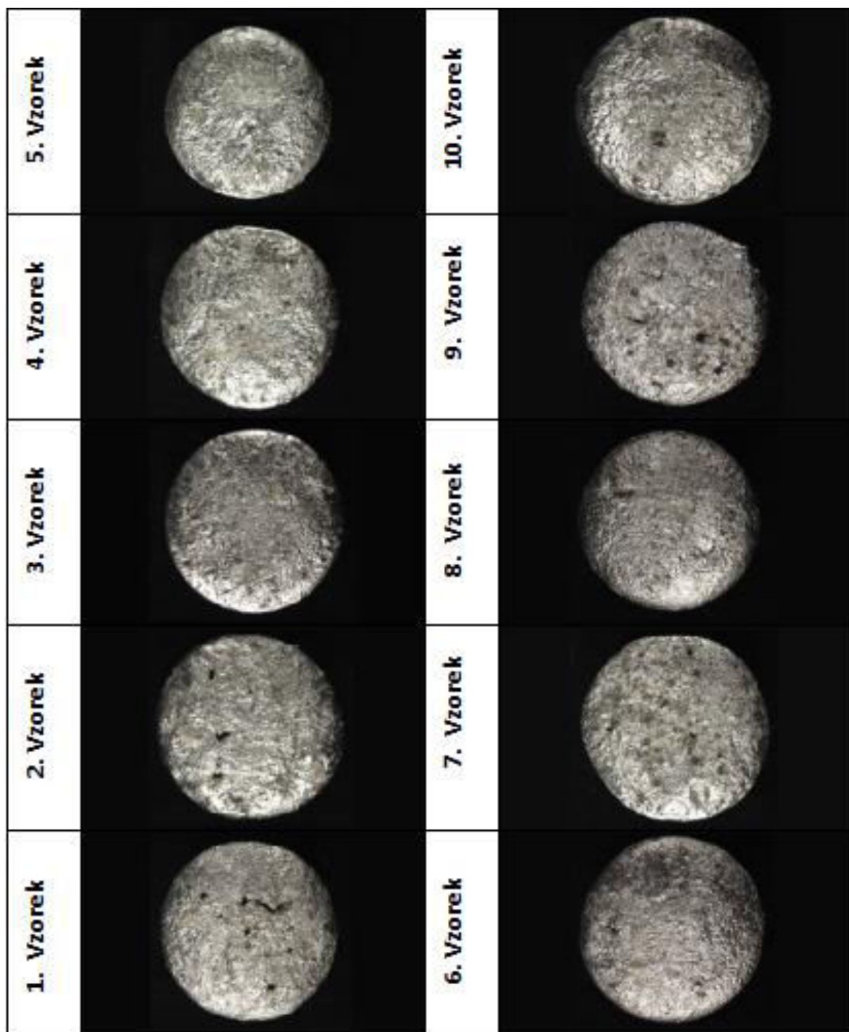
Příloha č. 1 Vzorčky ze slitiny EN AC-43 100 z materiálu o složení 60 % housky, 40 % vrat
