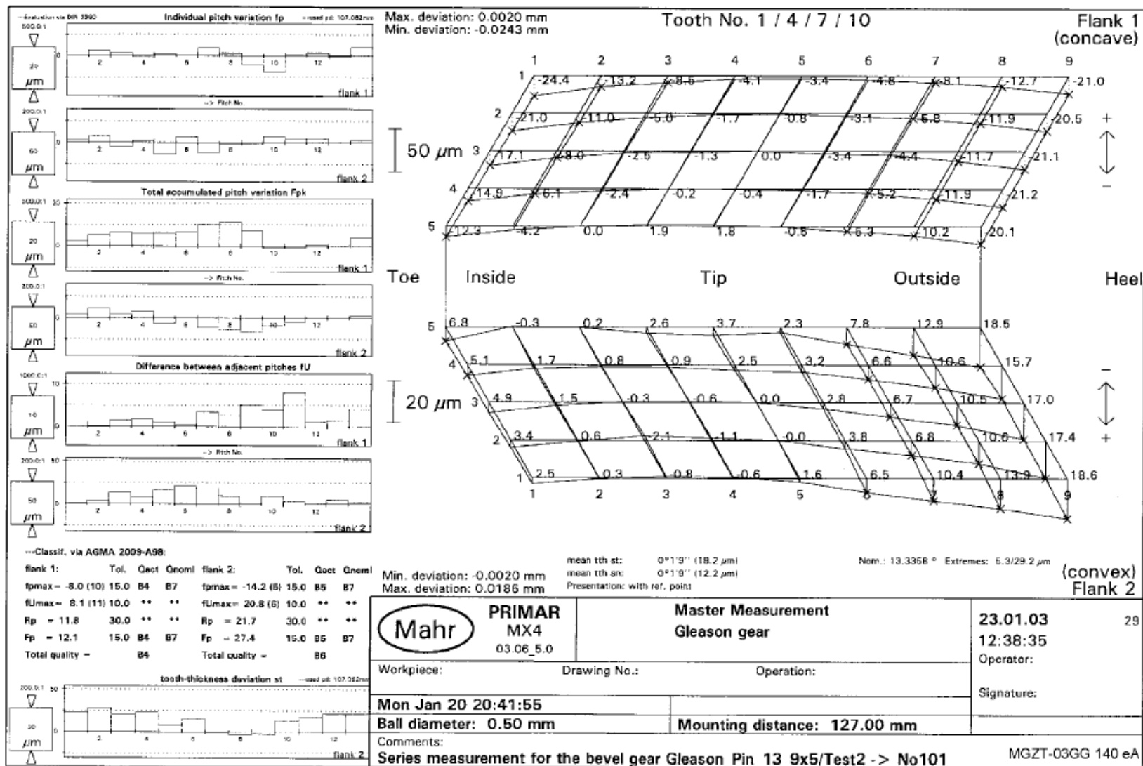
Příloha 5: Topografie ozubeného kola [24].
