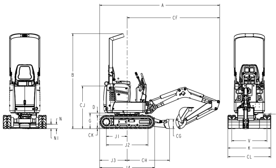
Obr.1 Základné rozmery stroja Bobcat E08
