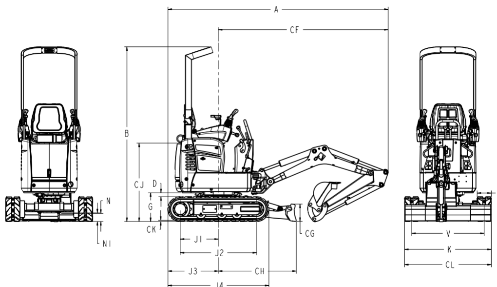
Obr.2 Základné rozmery stroja Bobcat E10
