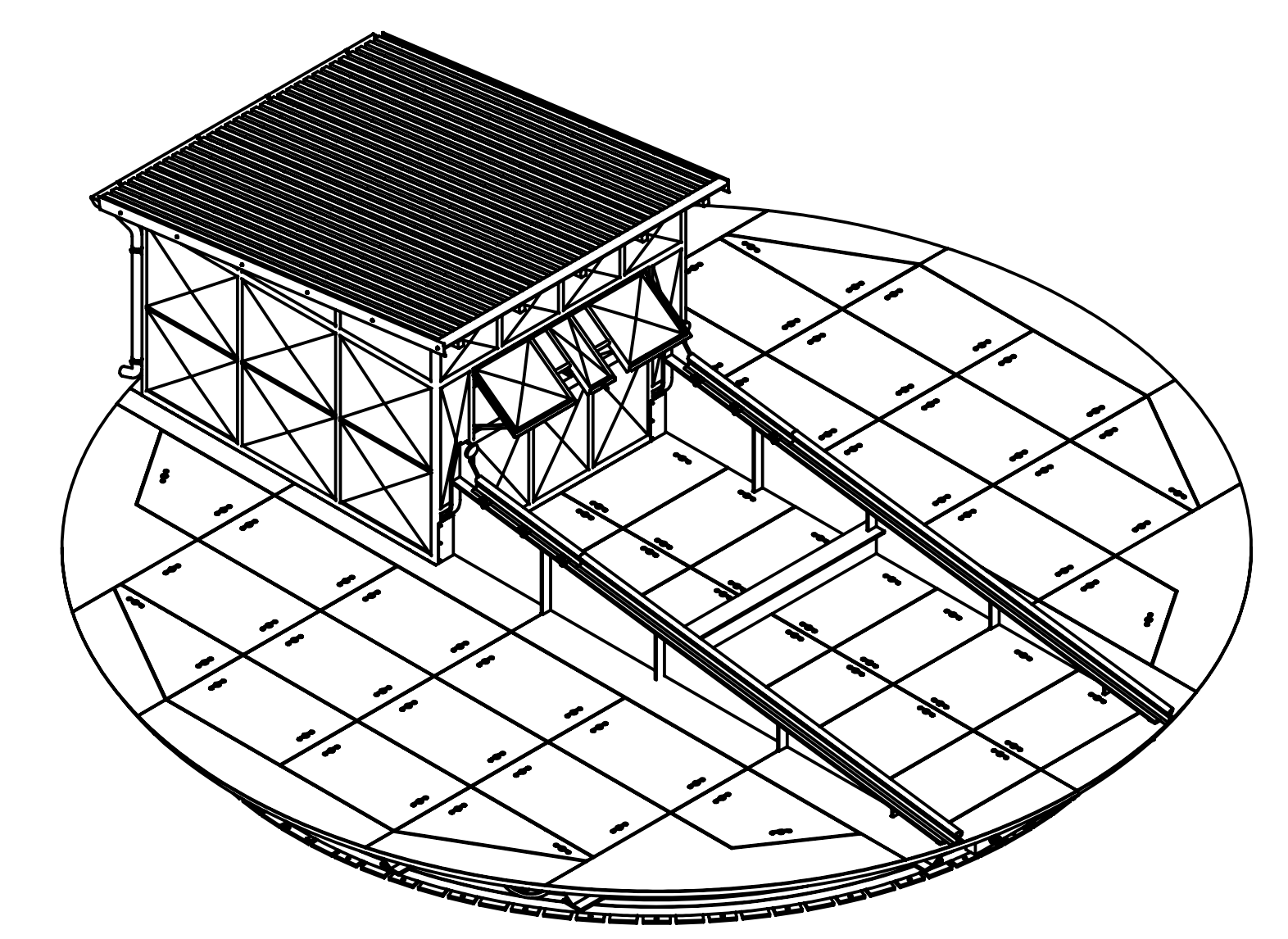
ISO (1:50)
