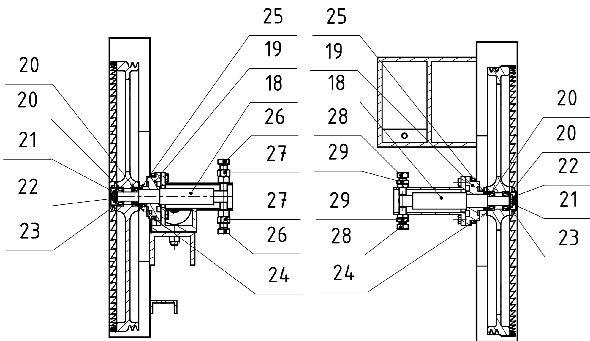
A-A (1:5)
