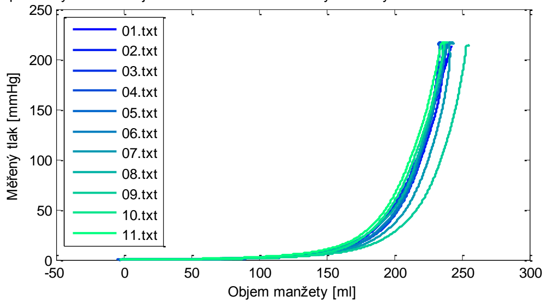
Opakovaný záznam objemově-tlakové charakteristiky manžety Omron HEM-CR24 22-32 nová
