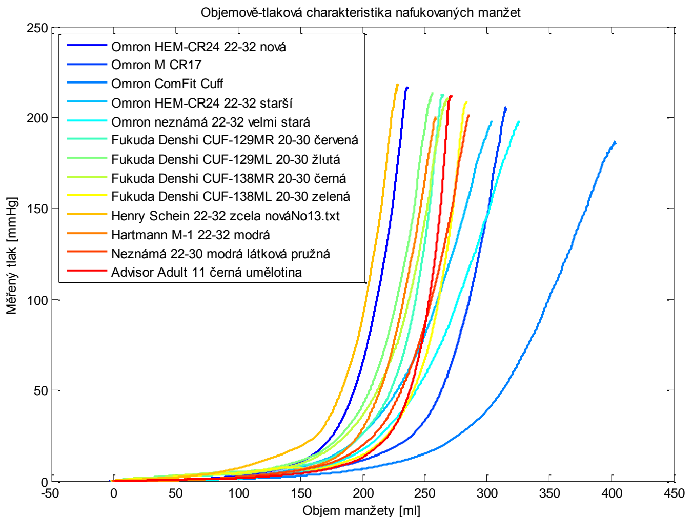
Graf 2 - Objemově-tlaková křivka pro celý soubor měřených manžet
