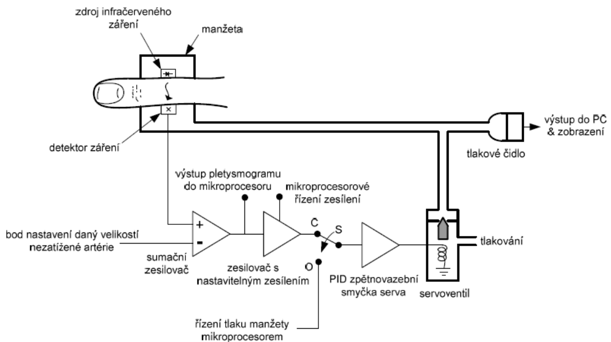
Obrázek 4 - Blokové schéma přístroje pro spojitě neinvazivní měření krevního tlaku. (8)
