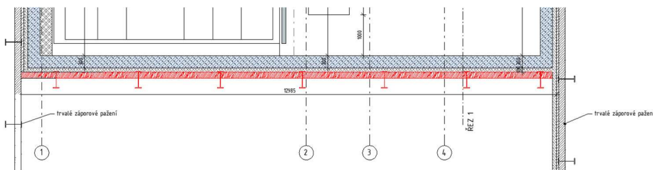
Obr. č.2 Výsek půdorysu 1.PP
