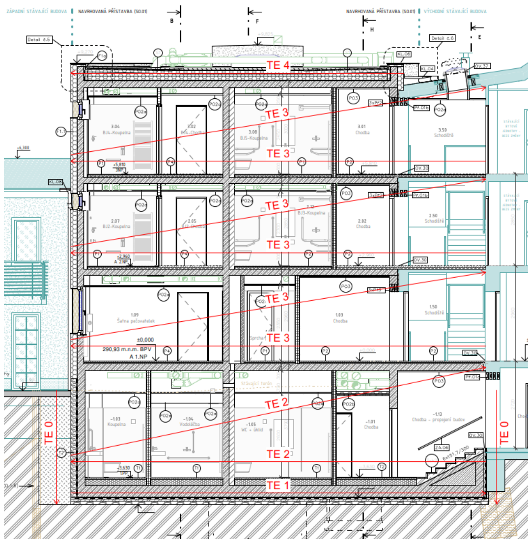
Obrázek 1: Technologické schéma TE 0 – 4, Interní soubor KONSIT a.s., Zpracoval: Ing. arch. Jan Řeháček, Ing. Martin Zlesák
