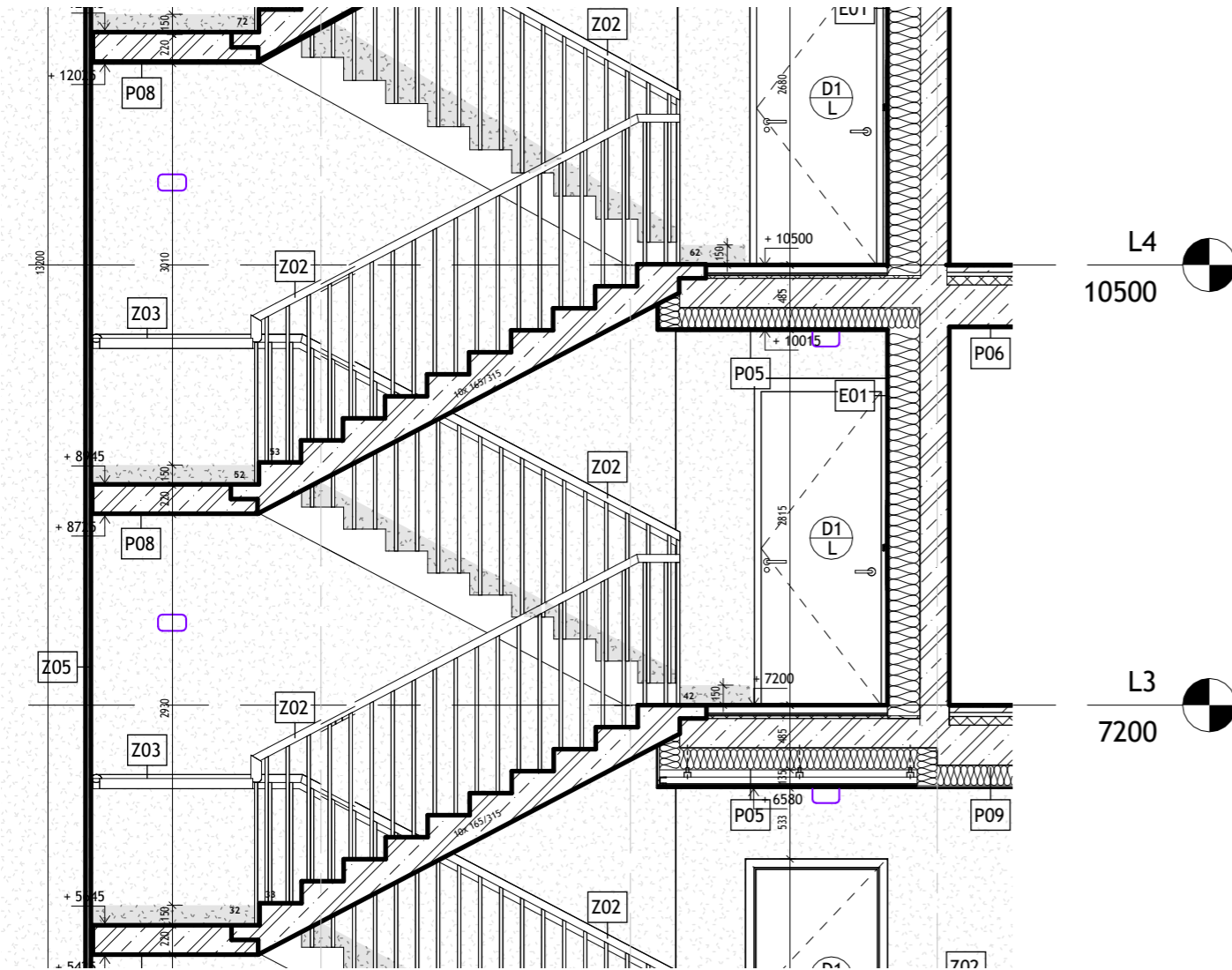
REZOPOHLAD C-C'
