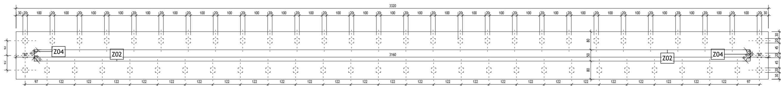
PÔDORYS ZÁBRADLIA M1:10
