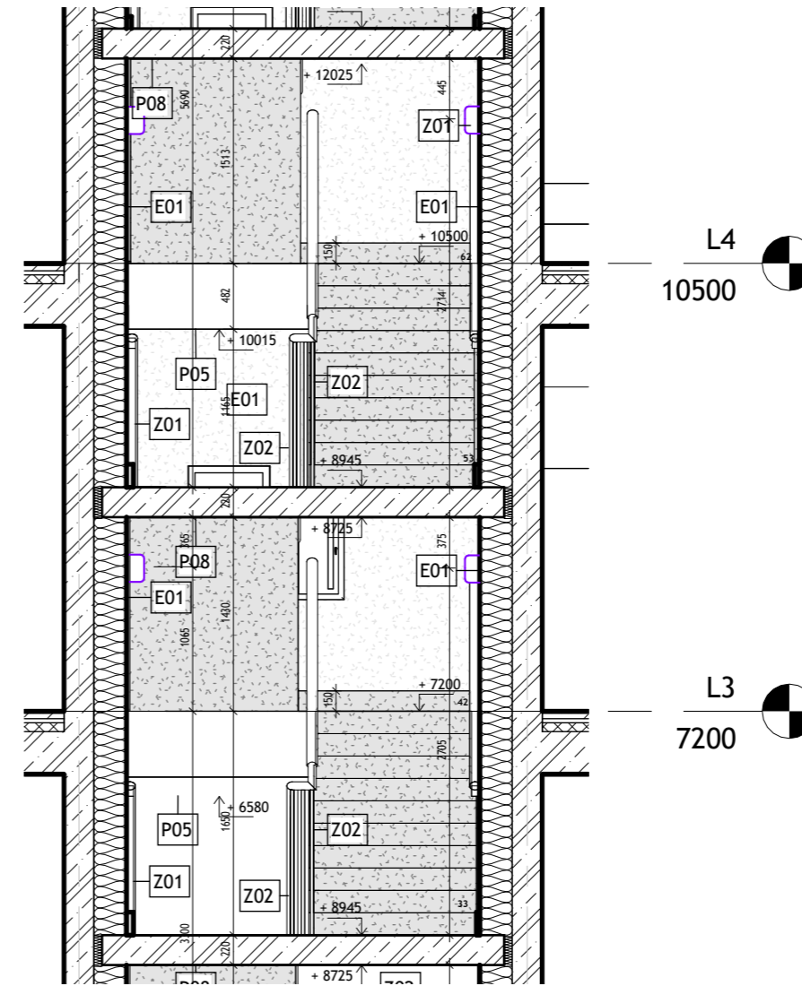
REZOPOHLAD D-D'
