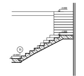
Uložení schodiště pohled na uložení nástupního ramene
