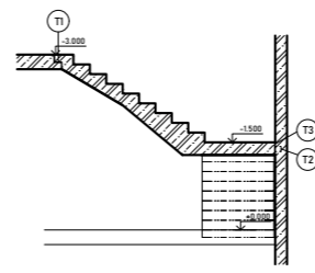
Uložení schodiště
