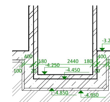
REZ A-A' - REZ VÝTAHOVOU ŠACHTOU, M 1:100
