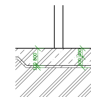
REZ B-B' - REZ STĽPOM, M 1:100
