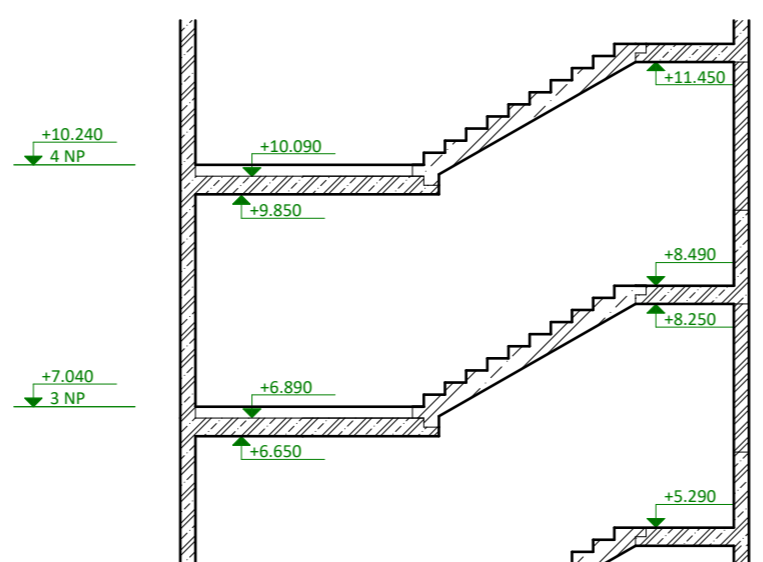
REZ B-B', M 1:100
