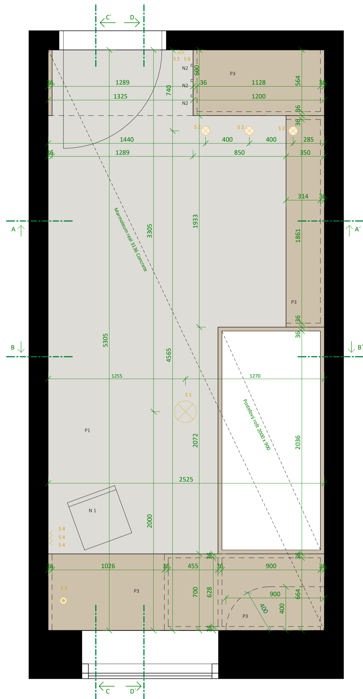
PŌDORYS - ŠTUDENTSKÁ IZBA
