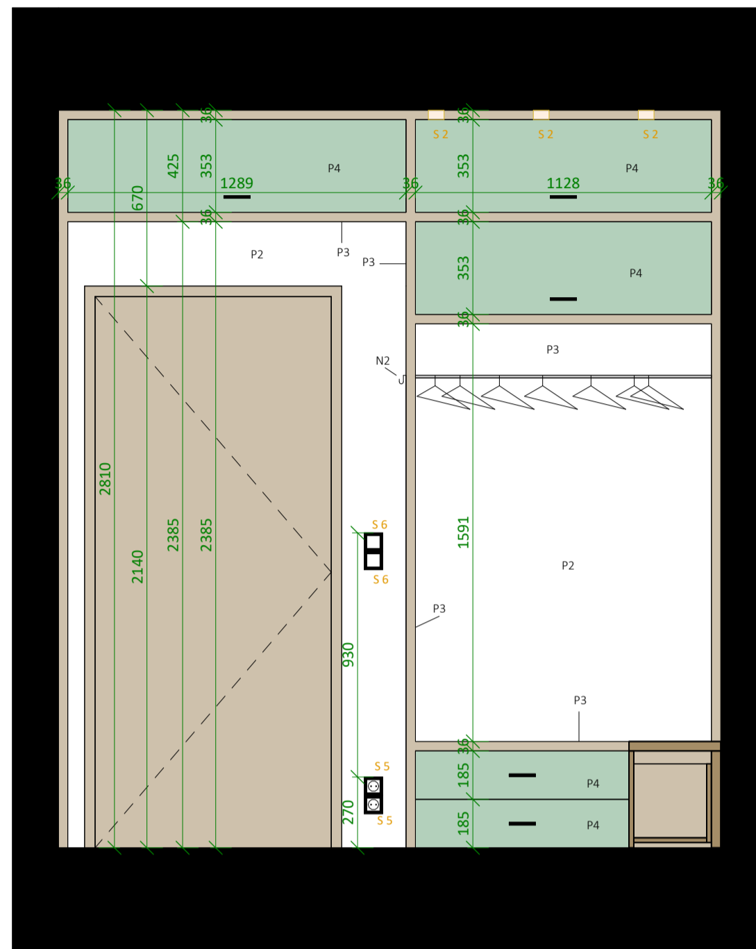
REZOPOHLAD A-A'
