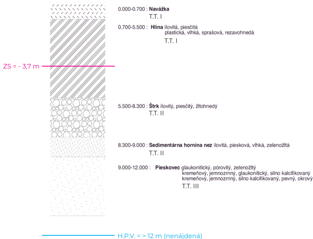
Obr. 2 - Geologický profil z vrtu 553261
