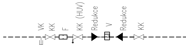
Vodoměrná sestava
