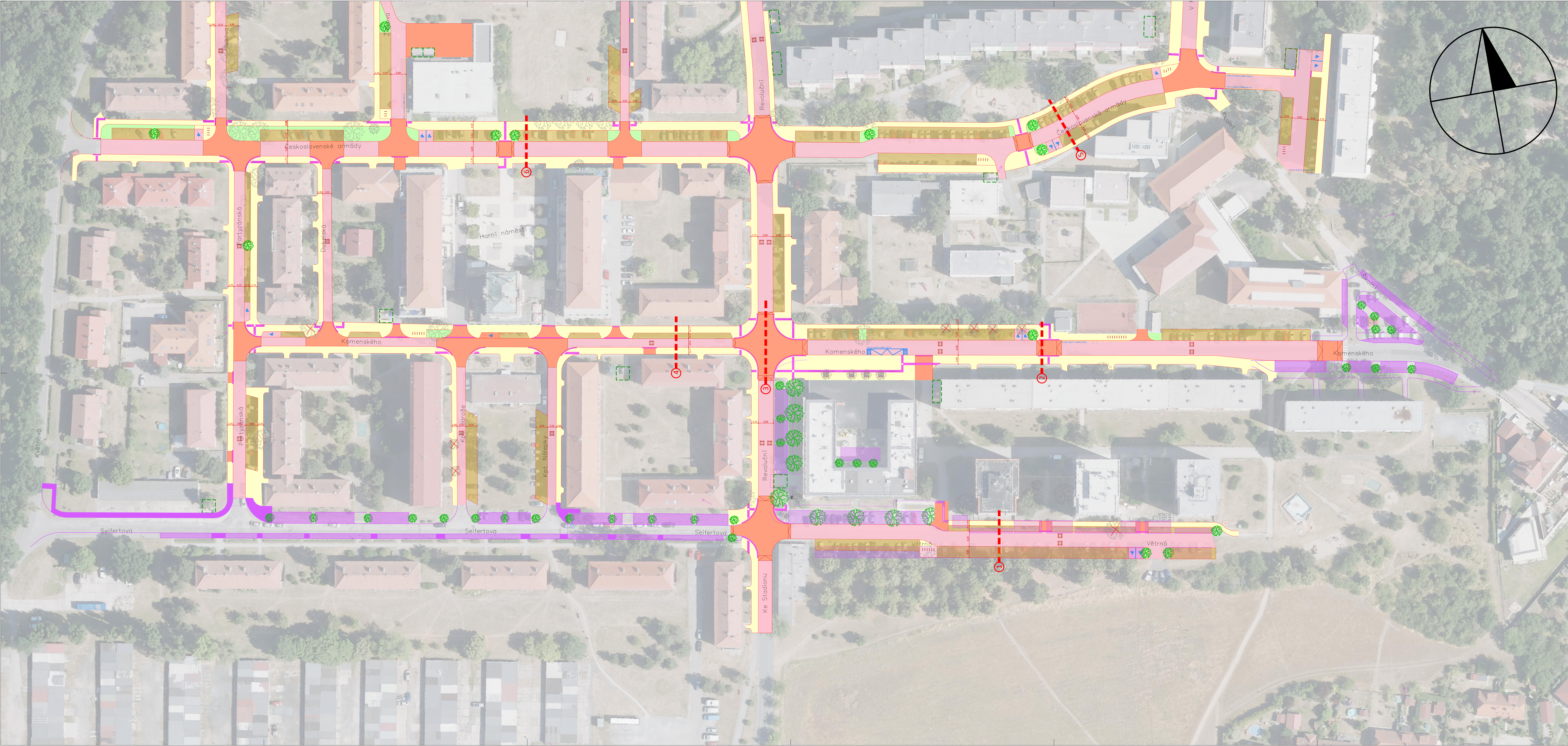
Situční výkres 1
