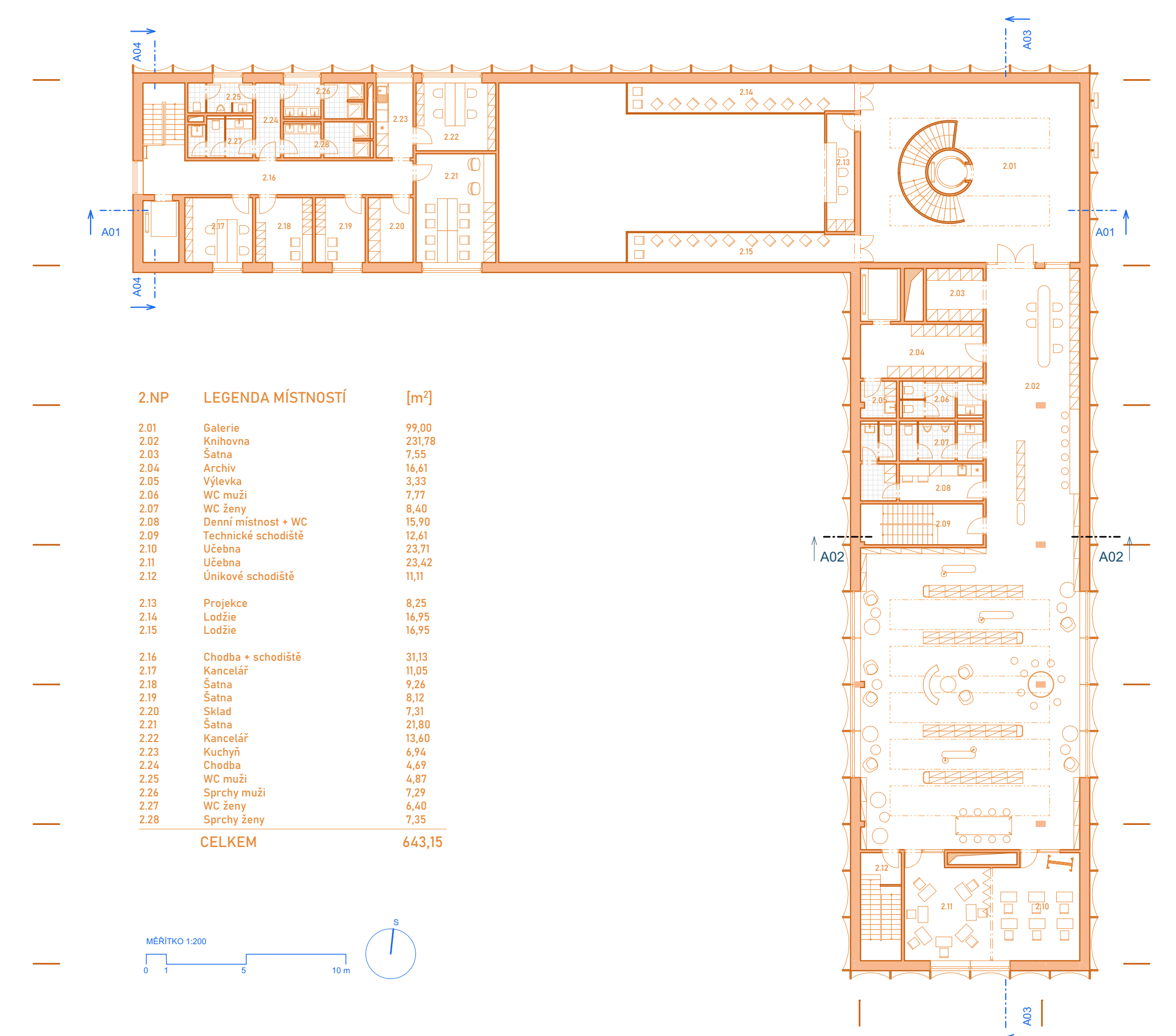
Půdorys 2.NP
