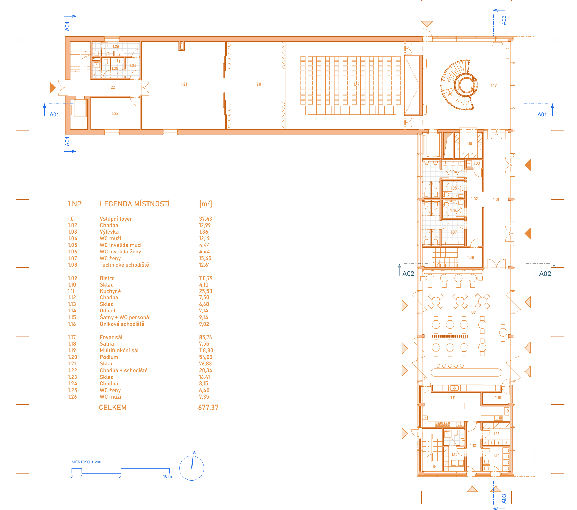
Půdorys 1.NP
