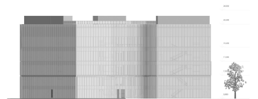
VÝCHODNÍ FASÁDA M 1:500
