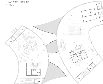
1. NADZEMNÍ PODLAŽÍ M 1:500
