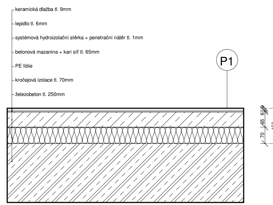
P1: SKLADBA PODLAHY - BISTRO
