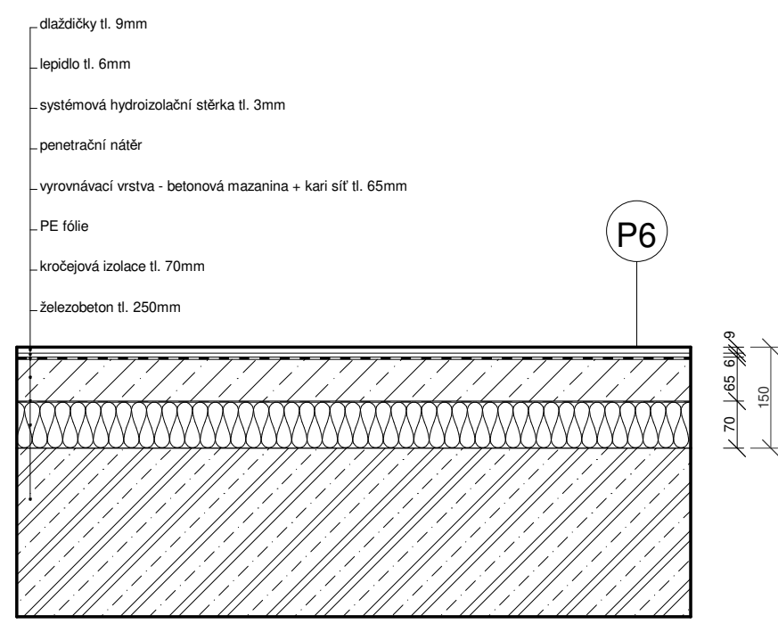
P6: SKLADBA PODLAHY - KOUPELNY 2NP, 3NP
