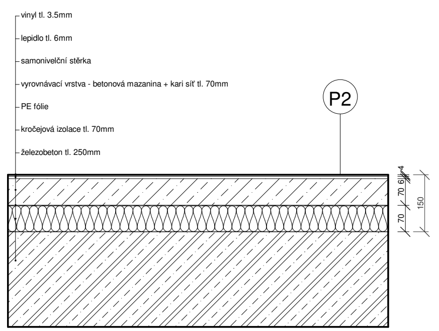
P2: SKLADBA PODLAHY - ZÁZEMÍ
