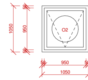
AUTOMATICKÝ OTEVÍRACÍ OKNO
