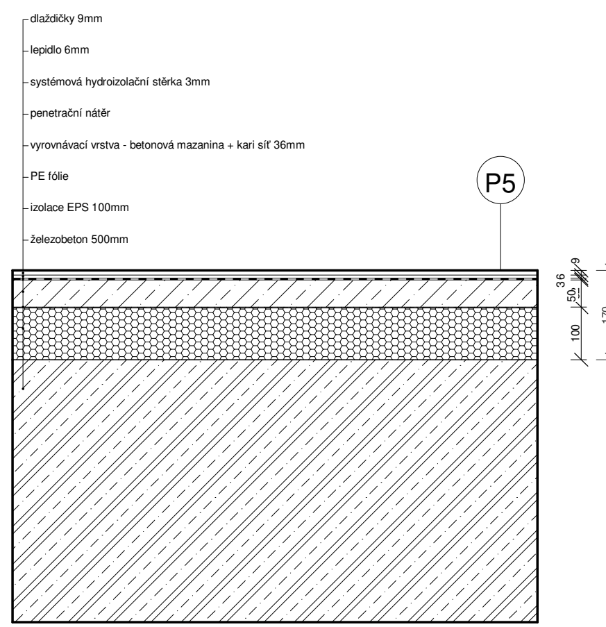
P5: SKLADBA PODLAHY - KOUPELNY 1NP
