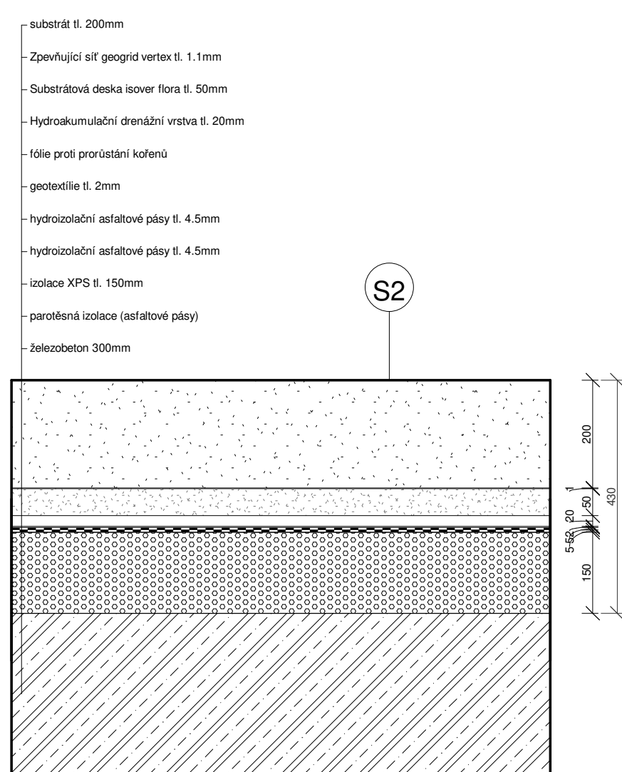
S2: SKLADBA STŘECHY - GARÁŽE
