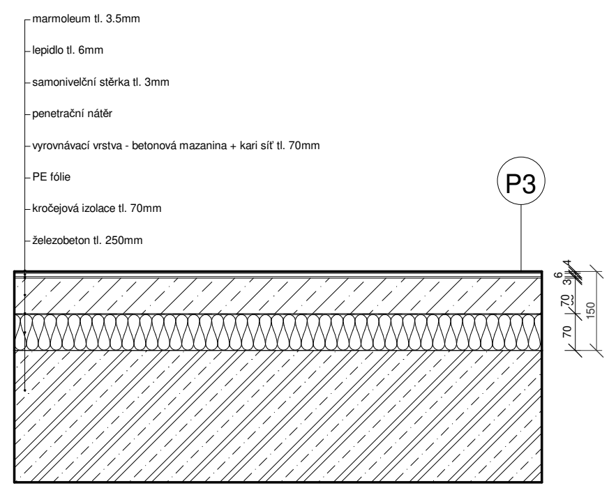
P3: SKLADBA PODLAHY - POKOJE 2NP, 3NP
