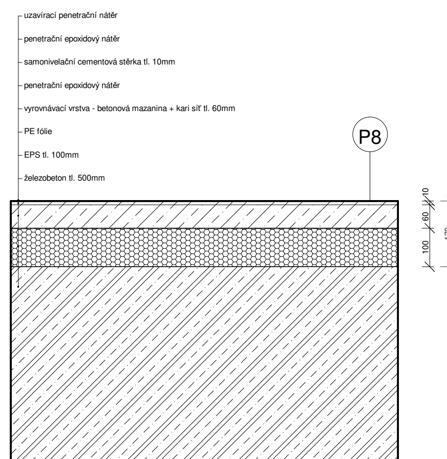
P8: SKLADBA PODLAHY - NÚC 1NP
