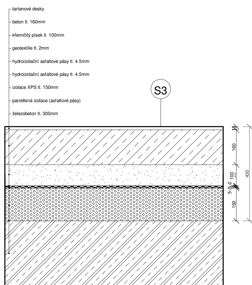
S3: SKLADBA STŘECHY - GARÁŽE
