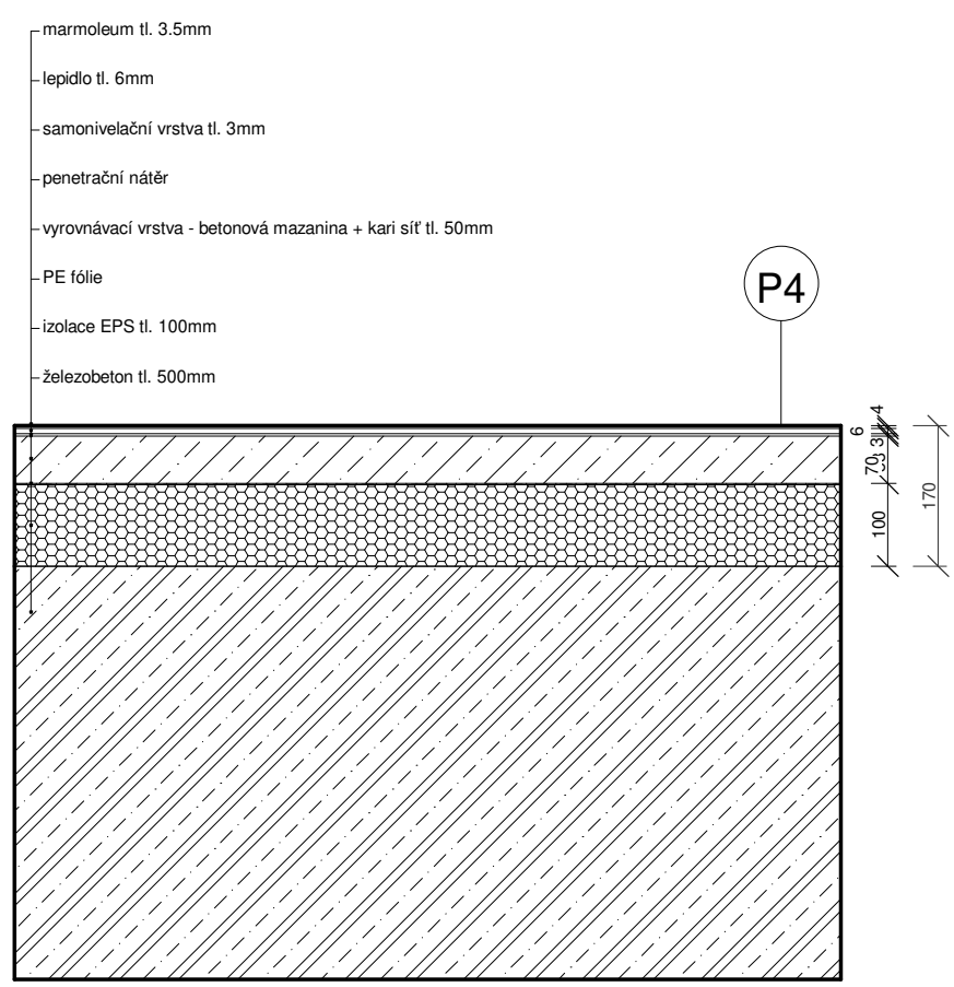
P4: SKLADBA PODLAHY - POKOJE 1NP
