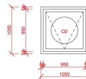
AUTOMATICKY OTEVÍRACÍ OKNO
